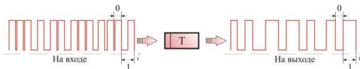
Рисунок 4.7 – Принцип работы триггера
