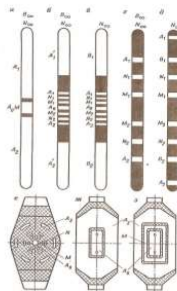
Зонды БК: а – 3-электродный (ТБК, АБК-Т, Э1); б – 7-электродный; в – 9-ти электродный псевдобоковой (БКС-2); г – дивергентный; д – дифференциально-дивергентный. Микрозонды: е – 4-электродный; ж – 2-электродный; з – 3-электродный
