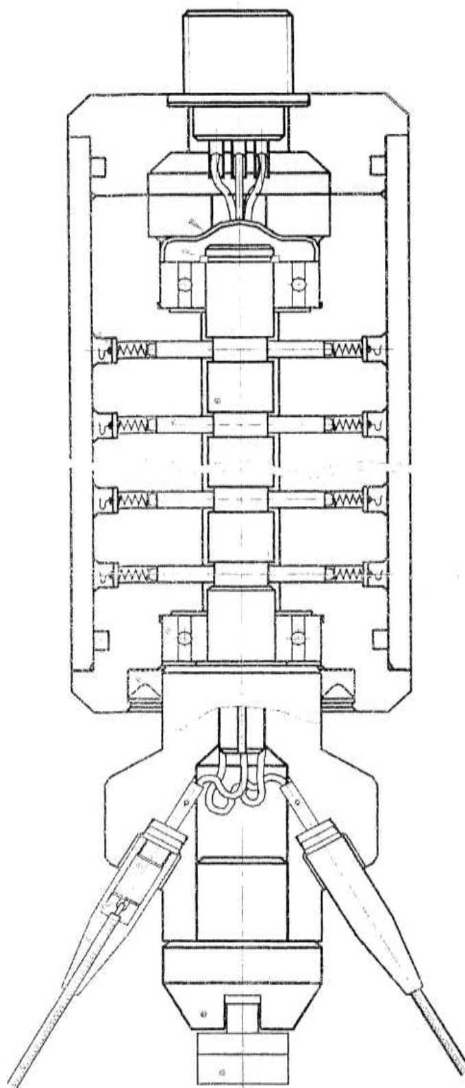
Рисунок 12.1 – Общий вид геофизического коллектора
