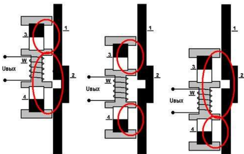
Рисунок 10.3 - Схема формирования сигнала локатора муфт
