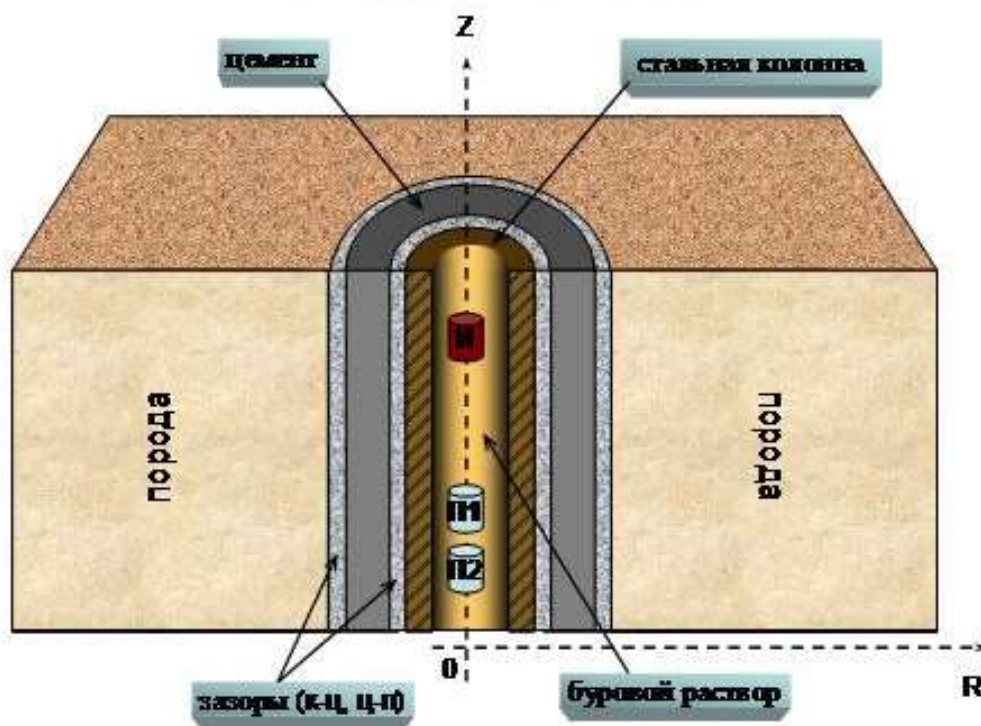
Рисунок 6.6 - Схема акустической цементометрии
