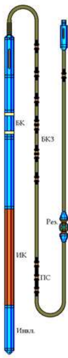
Рисунок 2.4—Общий вид комплексного прибора ЭК
