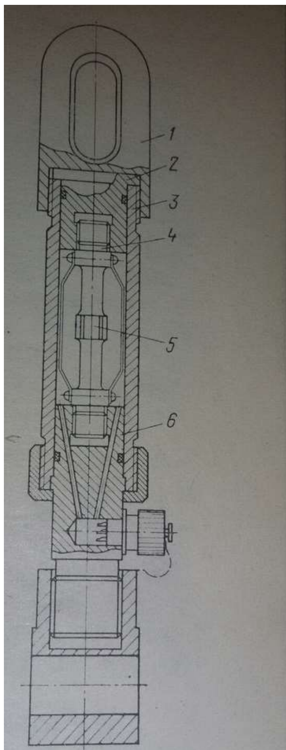
Рисунок 12.5 – Датчик натяжения кабеля
