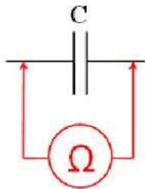
Рисунок 1.10 – проверка конденсатора методом заряд/разряд
