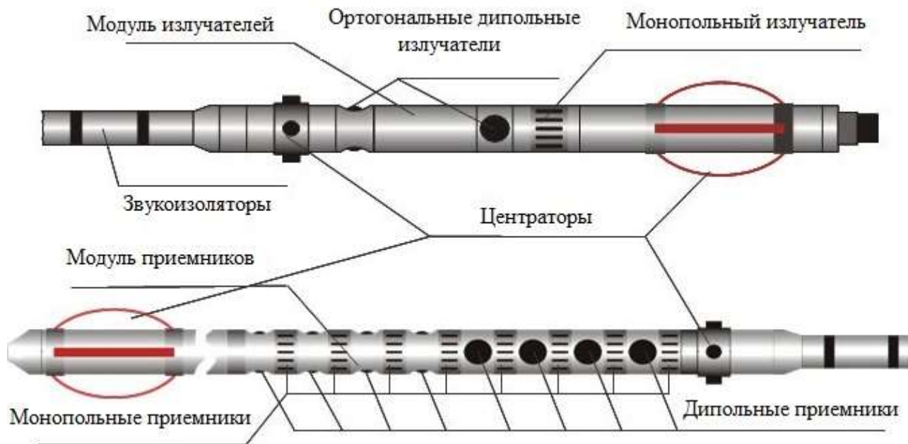
Рисунок 7.2 - Аппаратура волнового акустического каротажа ВАК-8
