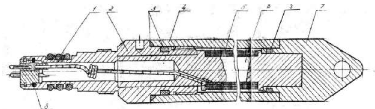
Рисунок 10.6 – Прихватоопределитель типа ПО
