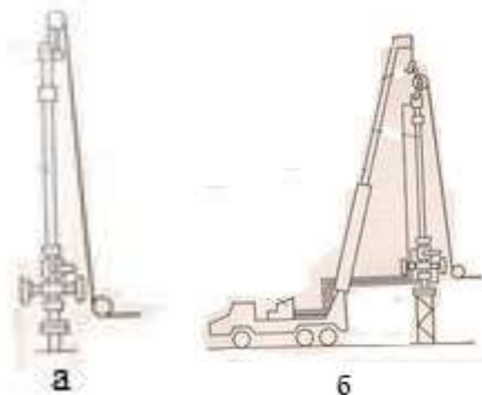
а - стационарный лубрикатор, б - лубрикатор установленный на передвижной вышке
