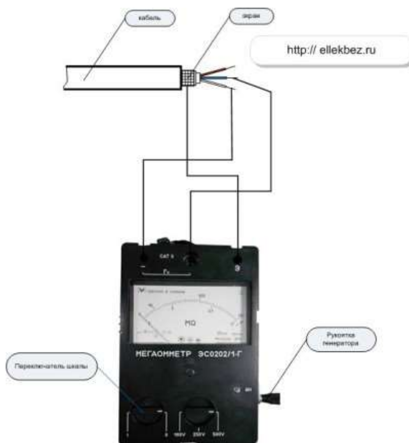
Рисунок 12.15 – Схема проверки изоляции жил кабеля
