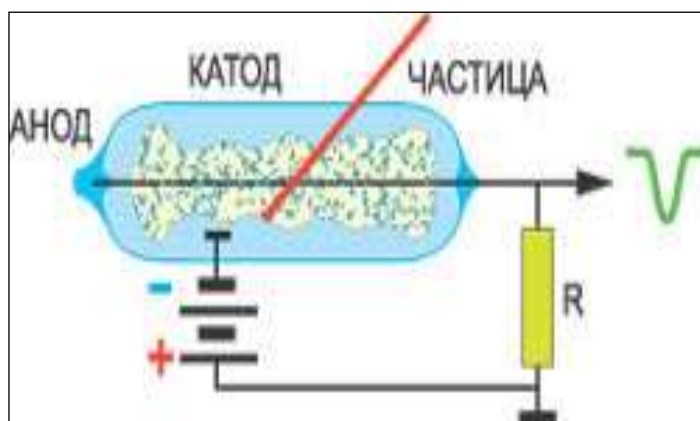
Рисунок 3.3 – Принципиальная схема газонаполненного детектора ионизирующего излучения
