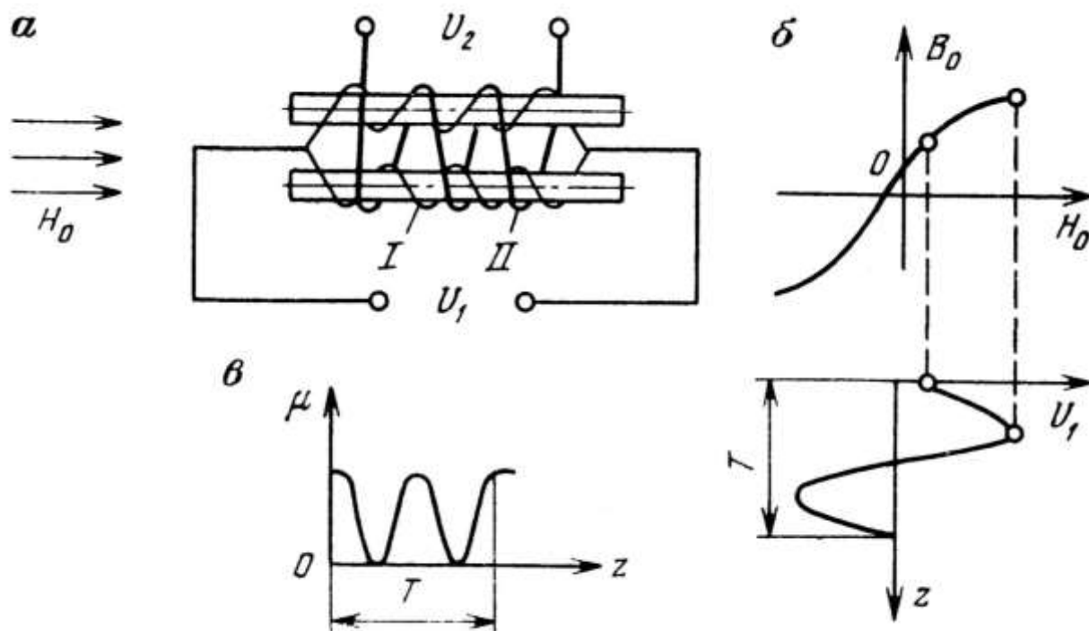
Рисунок 12.4 – Схема магнитомодуляционного меткоуловителя (а), характеристика B_0 = f(H_0) (б), кривая изменения магнитной проницаемости пермалловых стержней (в)
