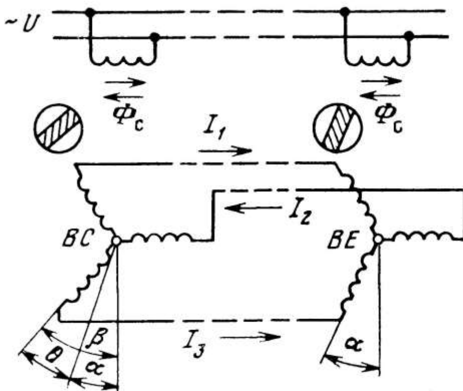
Рисунок 12.3 – Электрическая схема сельсинной передачи
