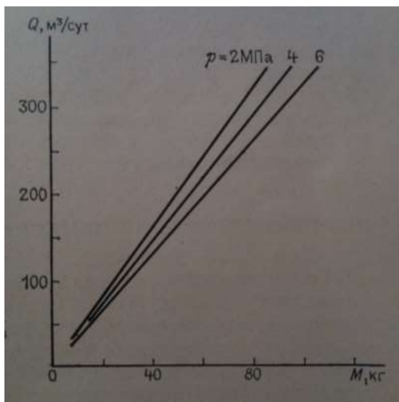
Рисунок 12.8 – График для определения массы груза M , необходимой для преодоления выталкивающей силы, действующей на кабель в зависимости от расхода жидкости Q
