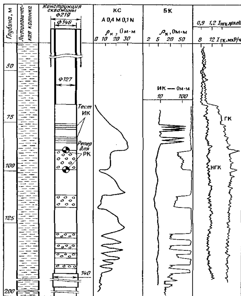
Рисунок 11.8 – Контрольная скважина с имитаторами физических свойств
