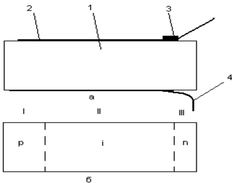
а – поверхностно-барьерный; б – с p-i-n переходом 1 – n -кремний; 2 – тонкий слой золота; 3, 4 – электрические контакты
