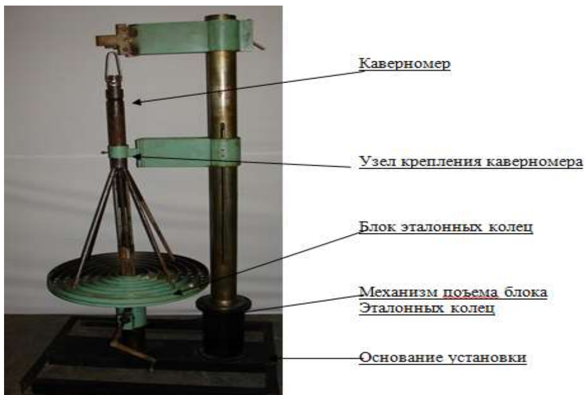
Рисунок 11.5– Общий вид установки УПК-1 для калибровки каверномеров
