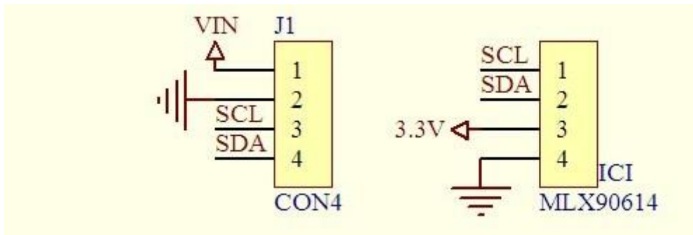
Рисунок 9– Подключение датчика в виде платы и собственно ИК датчика
