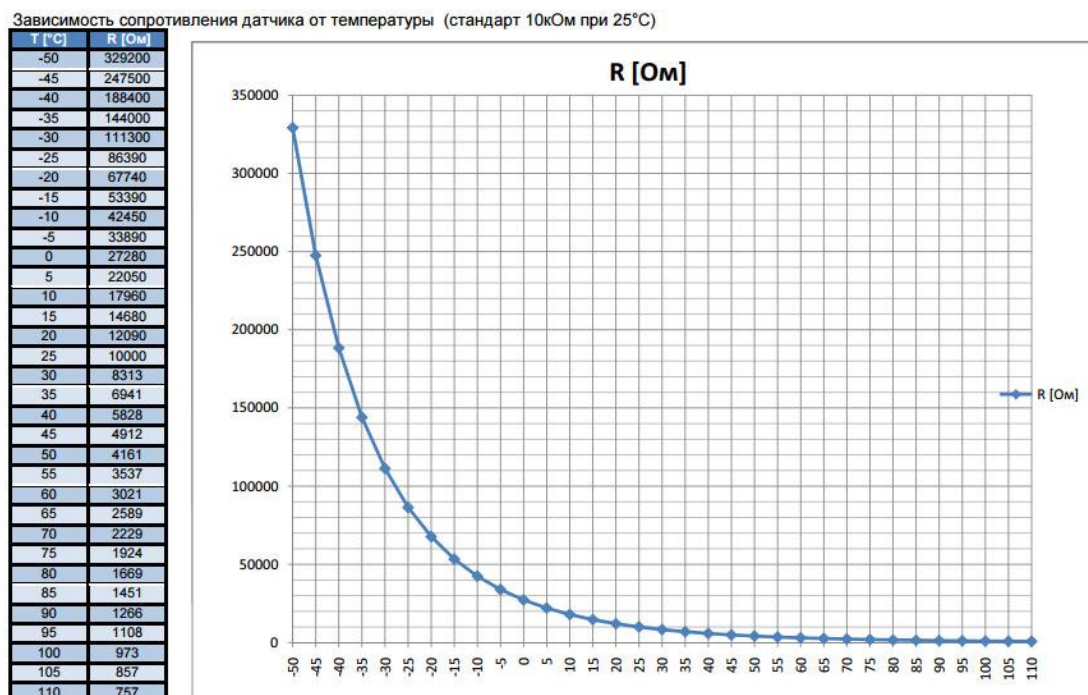
Рисунок 4 - Зависимость сопротивления датчика NTC-типа от температуры
