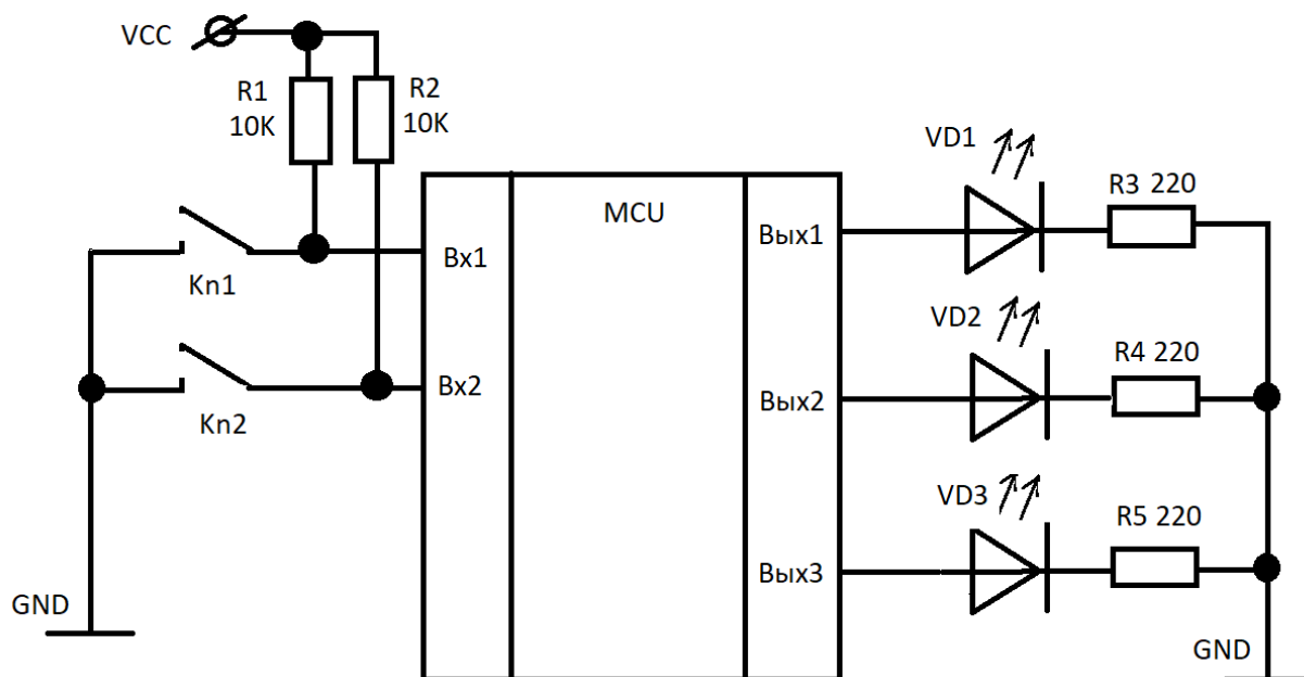
Рисунок 6- Электрическая схема устройства
