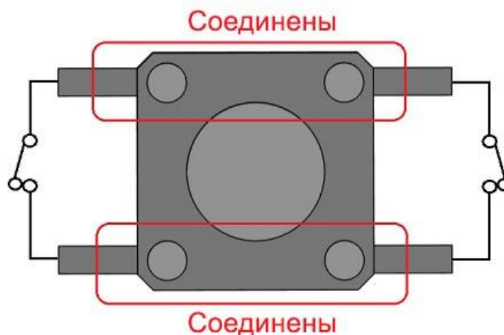
Рисунок 1 – Контакты кнопки из комплекта лабораторного оборудования
