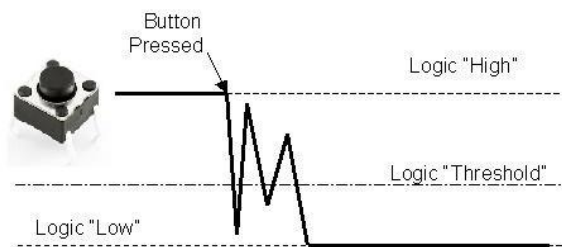
Рисунок 4 – Дребезг контакта при нажатии кнопки
