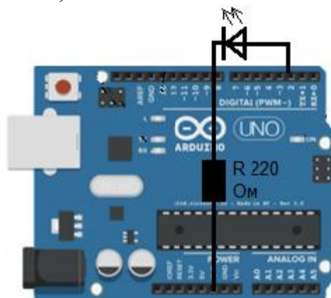
Рисунок 2 – Подключение светодиода
