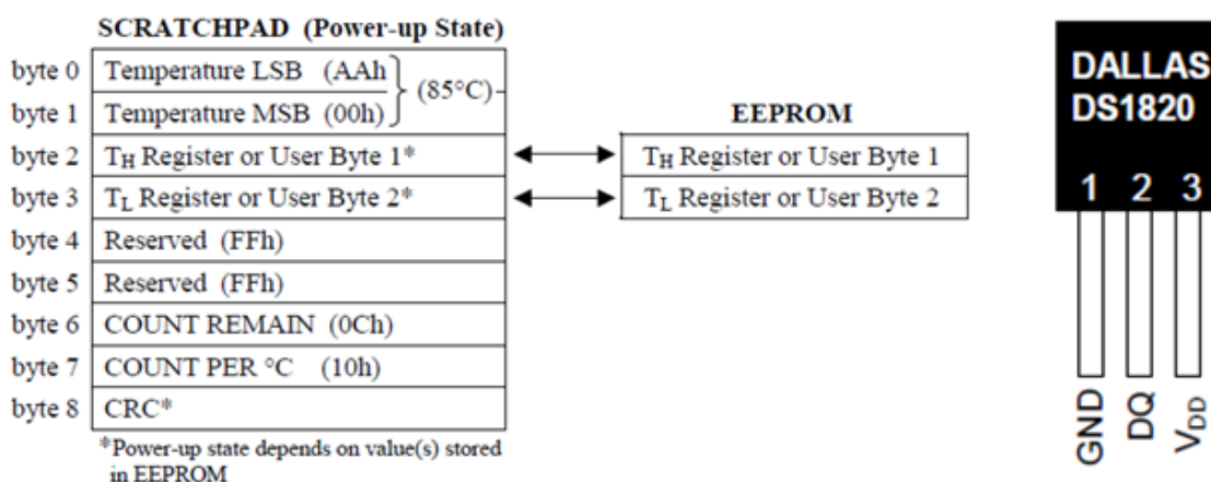
Рисунок 5 - Цифровой температурный датчик DS18B20
