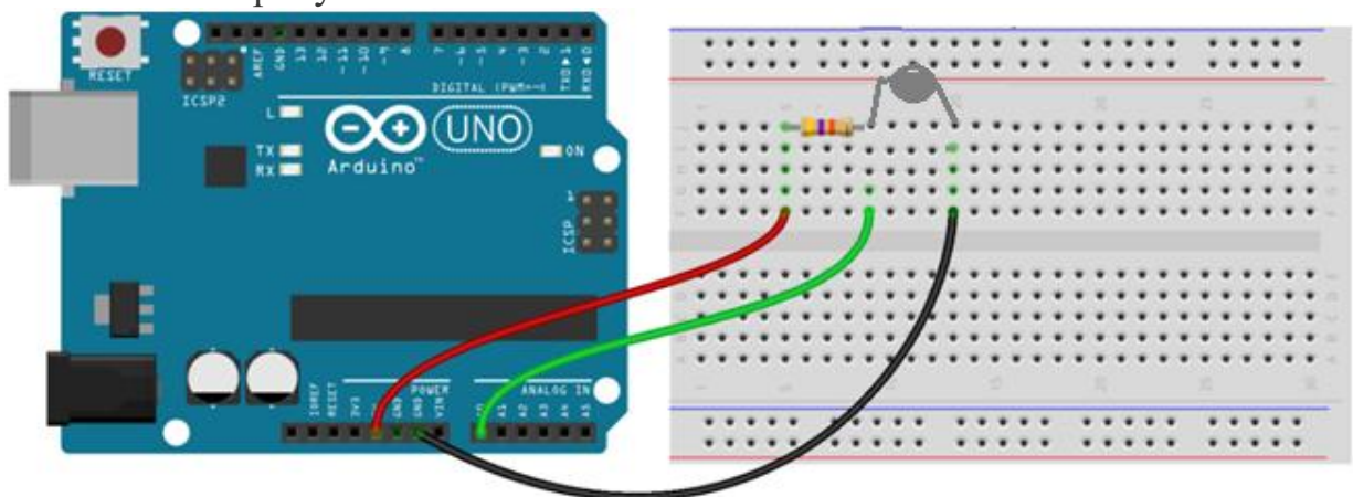
Рисунок 3 - Внешний вид макета
