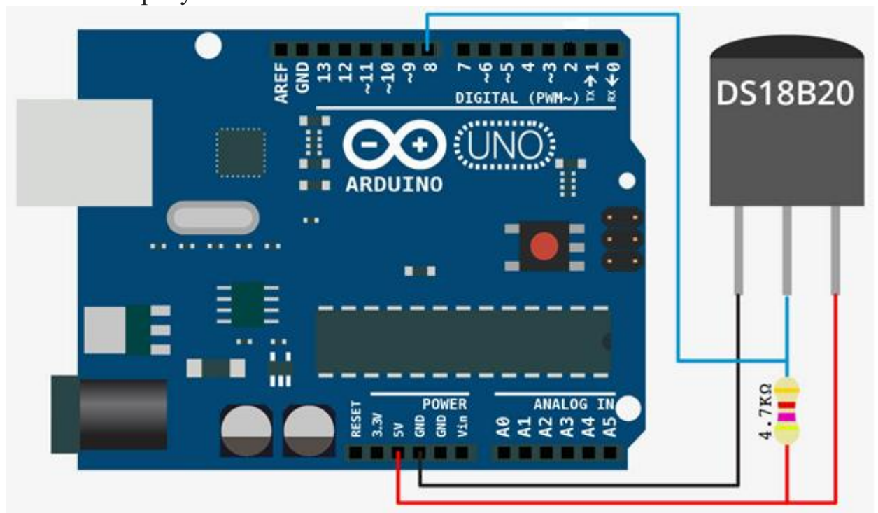
Рисунок 7 – Подключение датчика температуры к плате Arduino Uno
