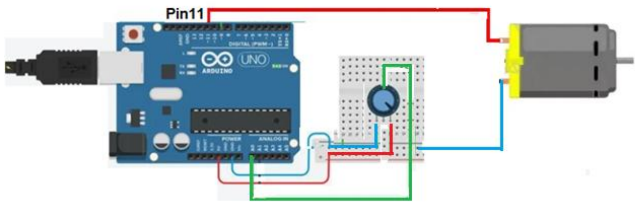
Рисунок 3 – Подключение электродвигателя постоянного тока, работающего от напряжения 3-5 В
