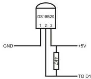
Рисунок 6 – Подключение датчика
