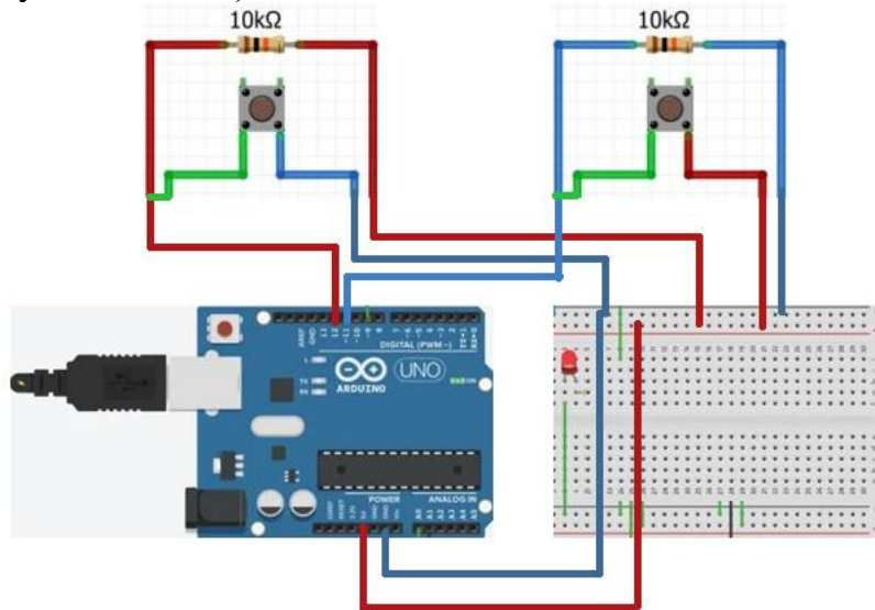
Рисунок 3 – Подключение кнопки с использованием внешних резисторов
