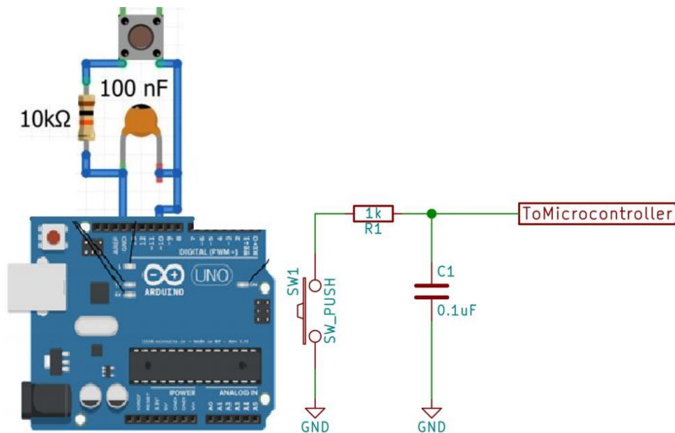
Рисунок 5- Защита от дребезга посредством RC-фильтра
