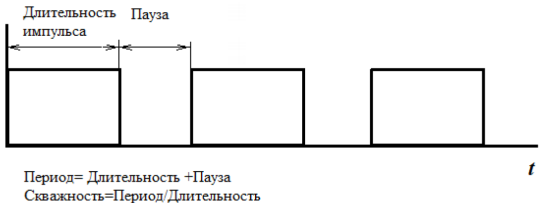
Рисунок 3 – Последовательность прямоугольных импульсов
