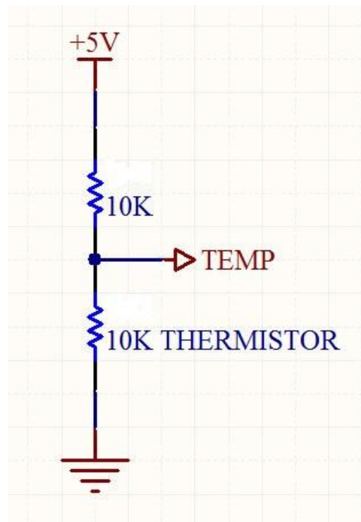
Рисунок 2 – Схема подключения термистора
