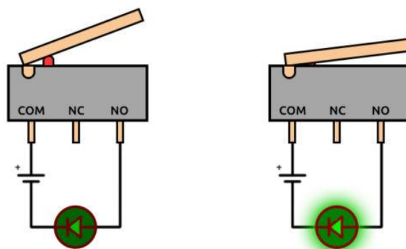
Рисунок 2 – Использование переключателя для управления светодиодом
