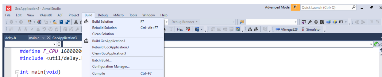
Рисунок 19 – Панель компилятора
