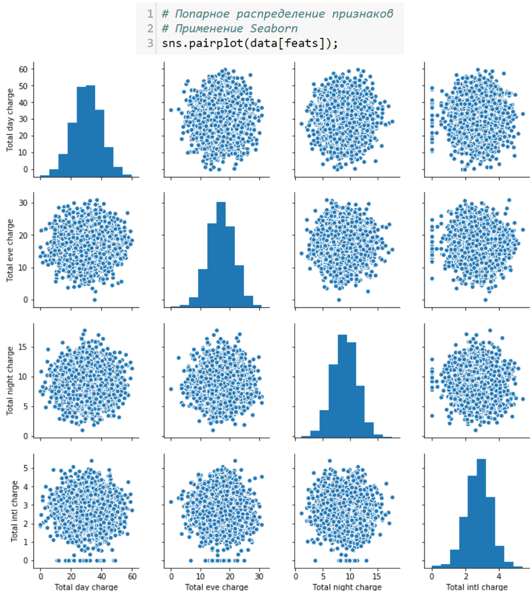
Рисунок 2.13 – Парное распределение признаков
