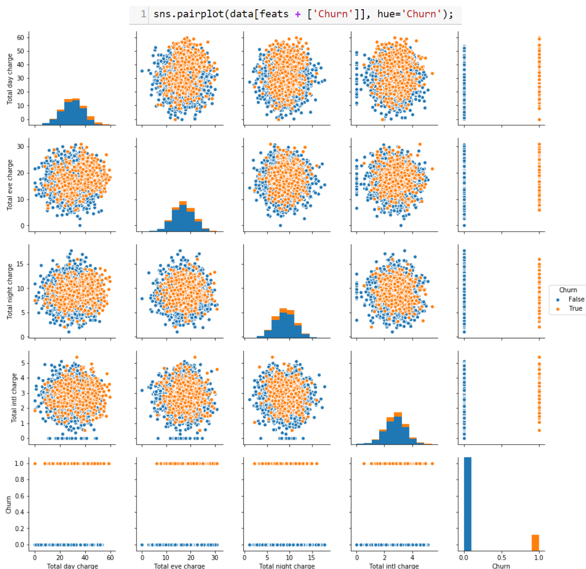
Рисунок 2.14 – Парное распределение признаков с визуализацией отказов
