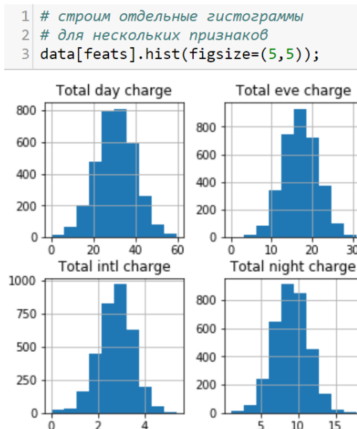
Рисунок 2.12 – Диаграммы для сравнения распределения числовых показателей
