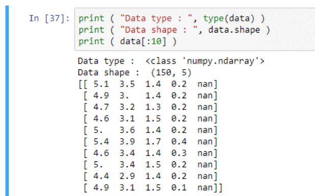
Рисунок 1.4 – Начальное исследование Iris.data
