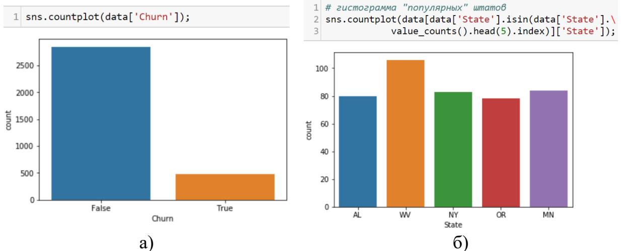
Рисунок 2.10 – График countplot : а) визуализация распределения признака Churn; б) визуализация пяти популярных штатов
