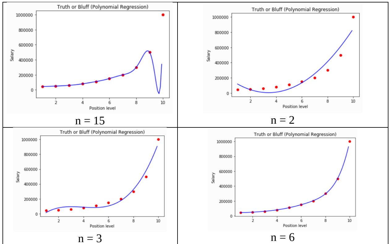
Рисунок 10.2 – Анализ модели полиномиальной регрессии
