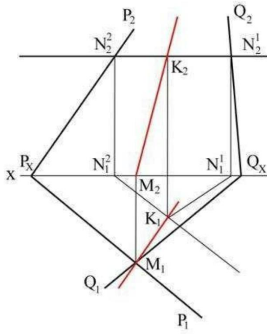
Рисунок 4.2 – Построение прямой пересечения плоскостей P и Q
