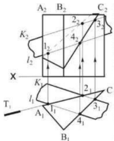
Рисунок 7.2 — Прямая призма (способ граней)
