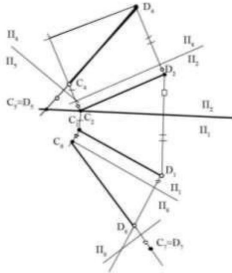
Рисунок 6.1 – Преобразования прямой
