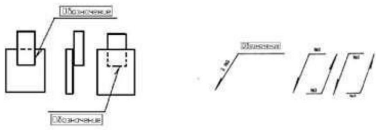
Рисунок 27.3 – Обозначение швов
