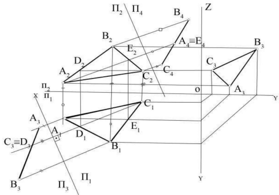
Рисунок 6.2 – Преобразования плоскости
