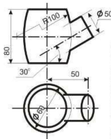
Рисунок— Тор (бочка) и цилиндр
