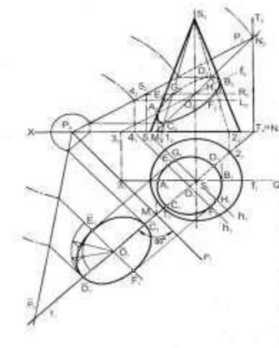
Рисунок 8.2. — Пересечение конуса плоскостью
