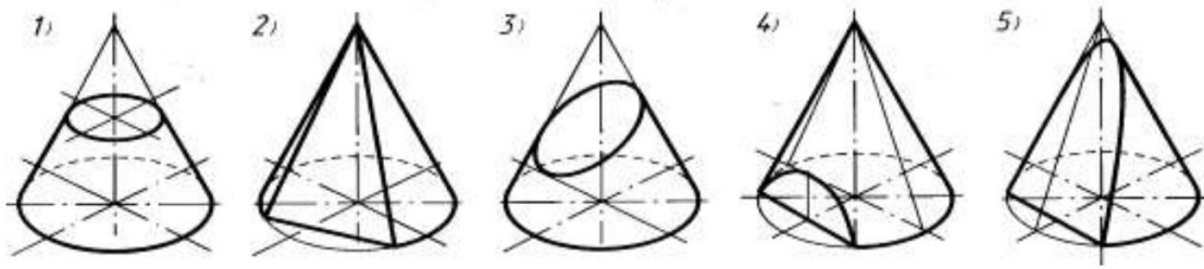
Рисунок 8.1. — Сечения конуса
