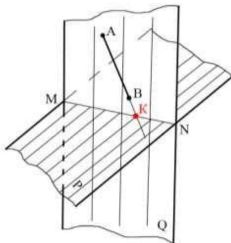
Рисунок 4.3 – Пересечение прямой АВ с плоскостью P
