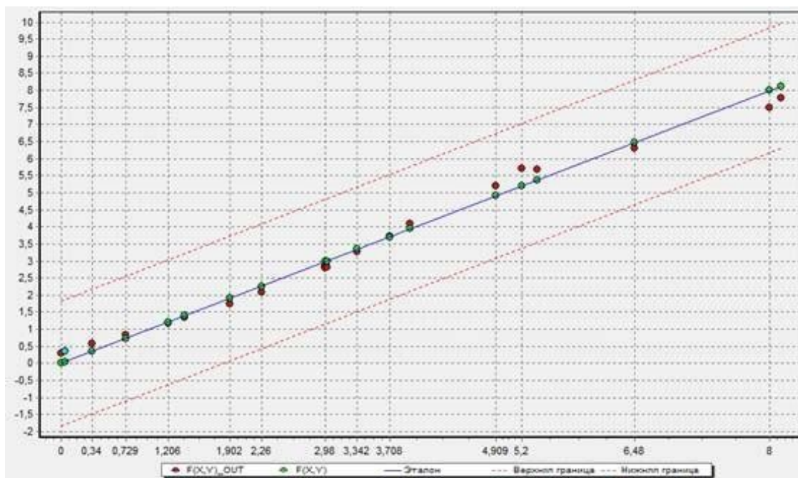
Рис. 2.12. Диаграмма рассеяния
