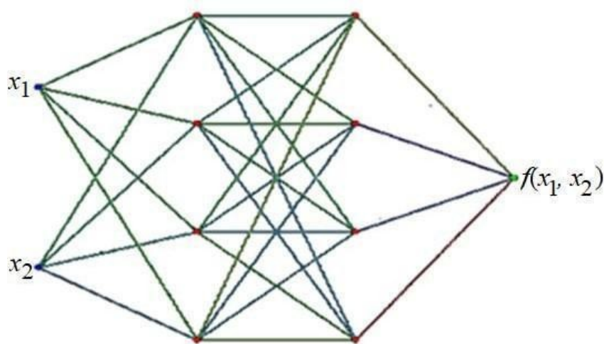
Рис. 2.11. Граф нейросети
