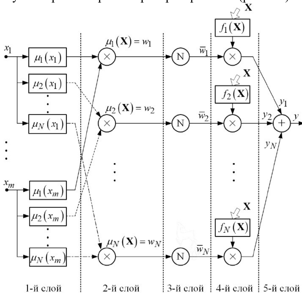
Рис. 4.2. Структура ANFIS -сети
