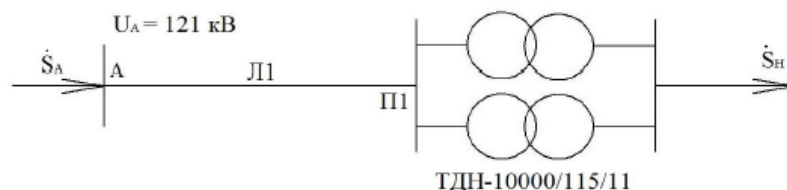
Рисунок 1 – Районная электрическая сеть
