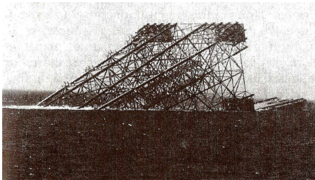
Рисунок 5 - Спуск стального каркаса платформы с помощью баржи
