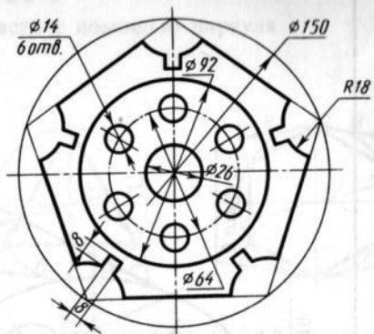
Крышка
