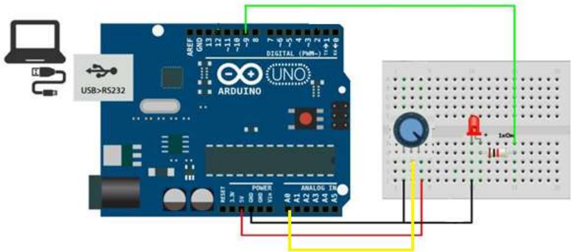
Рисунок 11 – Подключение внешних устройств
