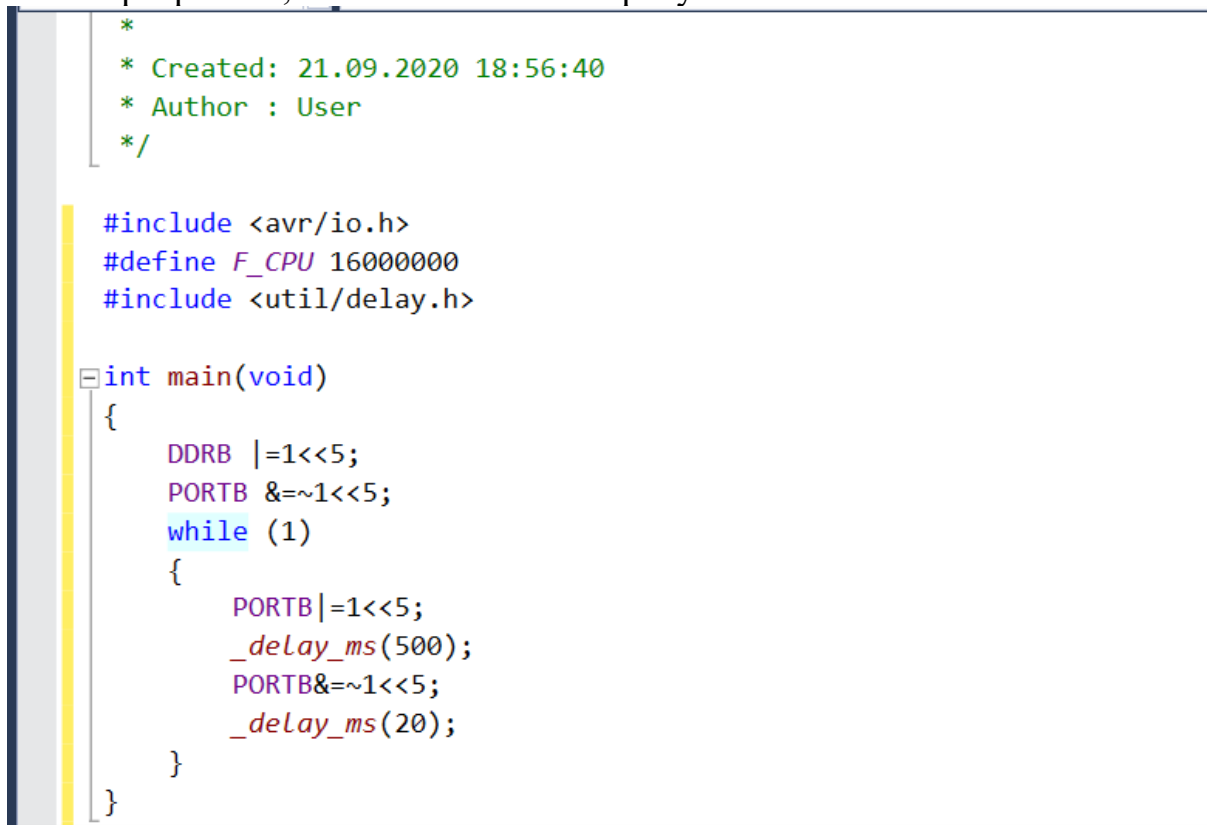
Рисунок 18 – Программа управления морганием светодиодом
