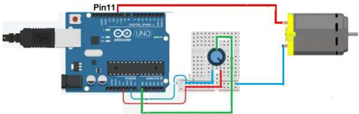
Рисунок 1 – Подключение электродвигателя постоянного тока, работающего от напряжения 3-5 В
