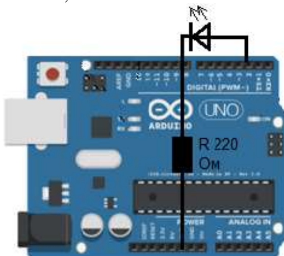
Рисунок 2 – Подключение светодиода
