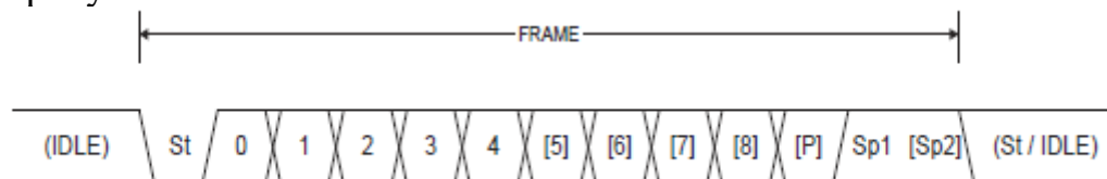
Рисунок 11 – Формат кадра USART
