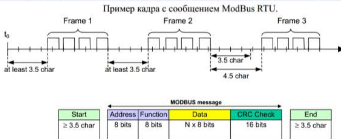
Рисунок 7 – Временная диаграмма передачи кадров в формате RTU
