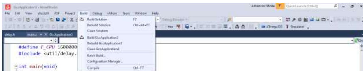
Рисунок 19 – Панель компилятора
