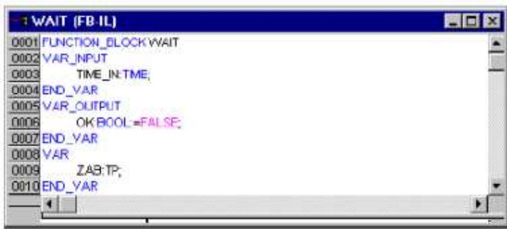
Рисунок 3 – Программирование "WAIT"
