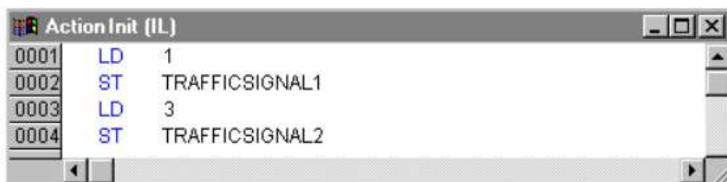
Рисунок 7- Этап Init
