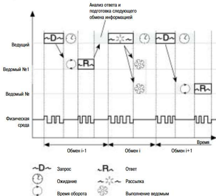
Рисунок 3 – Последовательность пересылки данных
