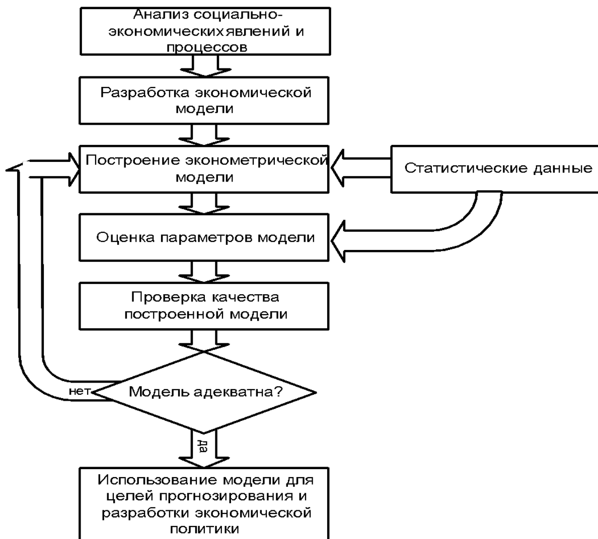
Рис. 1.2 Основные этапы эконометрического исследования
