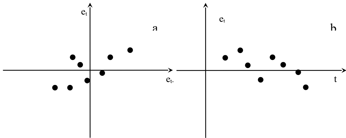
Рис. 12.8 Случаи, когда невозможно определить автокорреляцию при помощи графического метода
