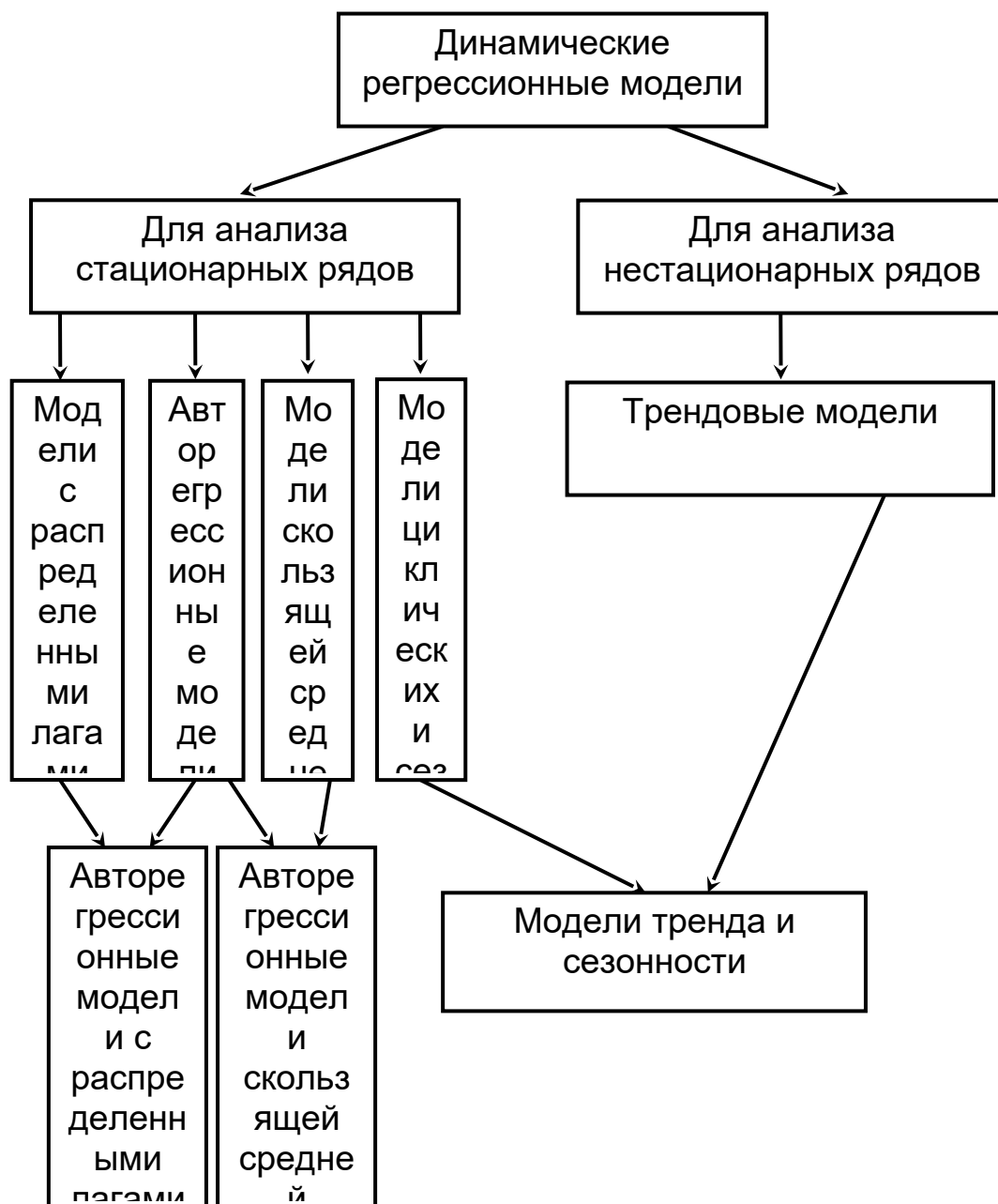
Рис. 11.1 Типология динамических регрессионных моделей
