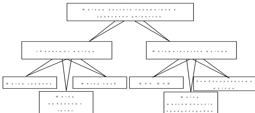
Рис. 5.1 Основные методы расчета коэффициентов регрессии
