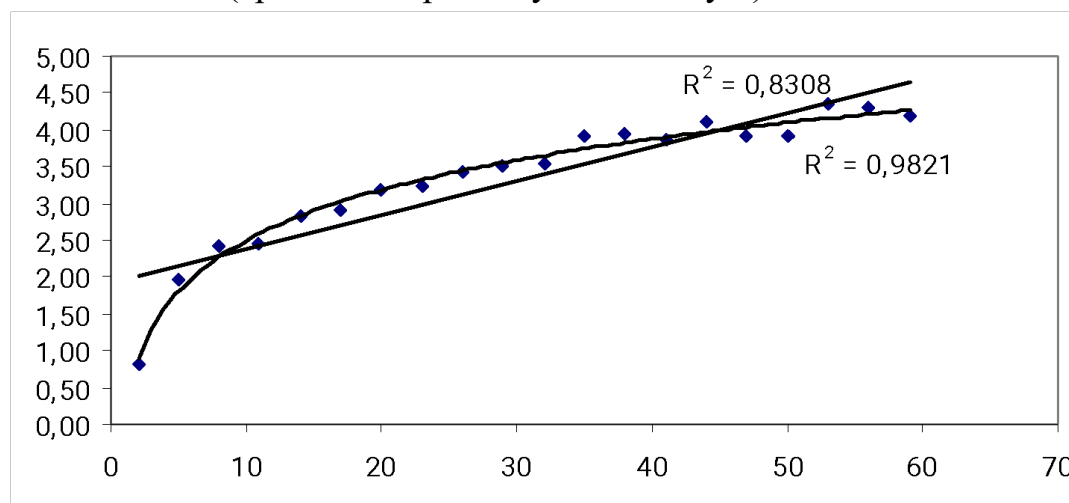
Рис. 12.10 Устранение автокорреляции изменением спецификации модели с линейной на логарифмическую
