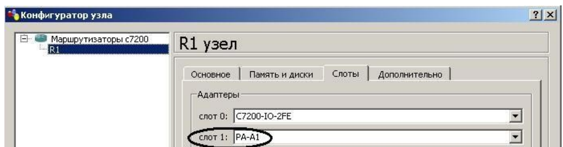
Рисунок 21 – окно «Конфигуратор узла» маршрутизатора
