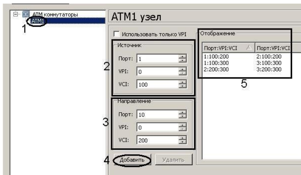
Рисунок 22 – окно «Конфигуратор узла» коммутатора ATM
