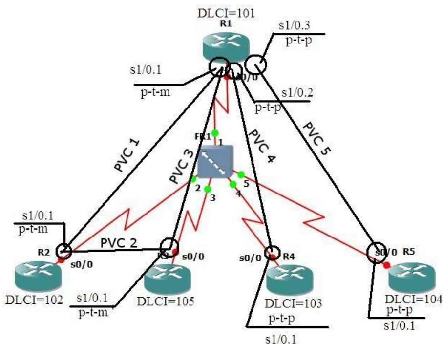
Рисунок 19 – Исследуемая топология
