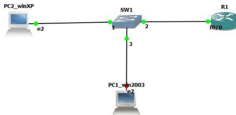
Рисунок 9 - PPPoE топология
