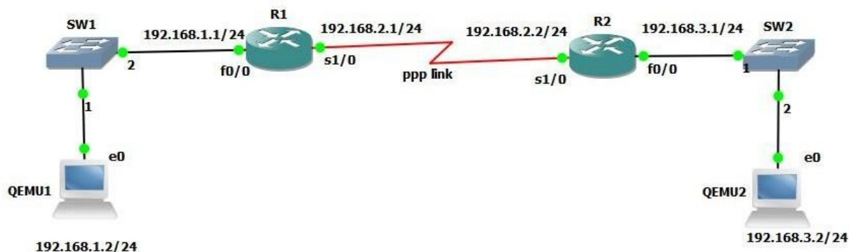
Рисунок 1 - Топология сети
