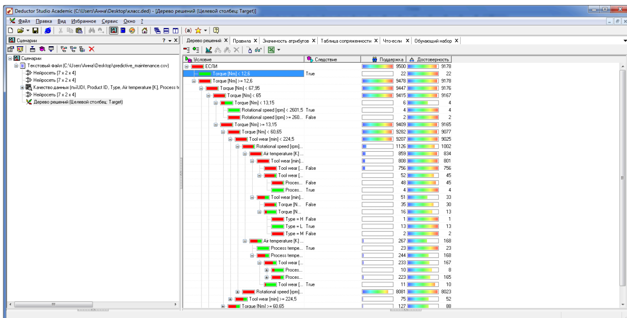
Рисунок 5 – Дерево решений
