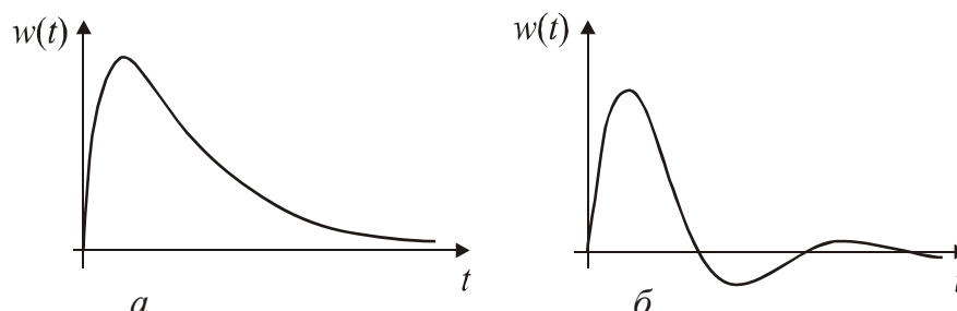
Рис. 3.2. Импульсные переходные функции системы второго порядка: a – с вещественными полюсами; b – с комплексно-сопряженными полюсами
