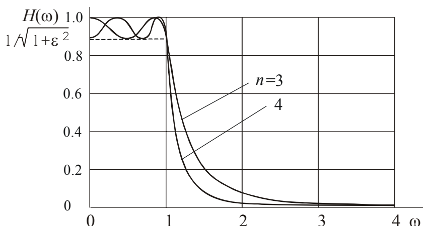
Рис. 6.2. АЧХ нормированных фильтров Чебышева первого типа ( \varepsilon = 0.765 )
