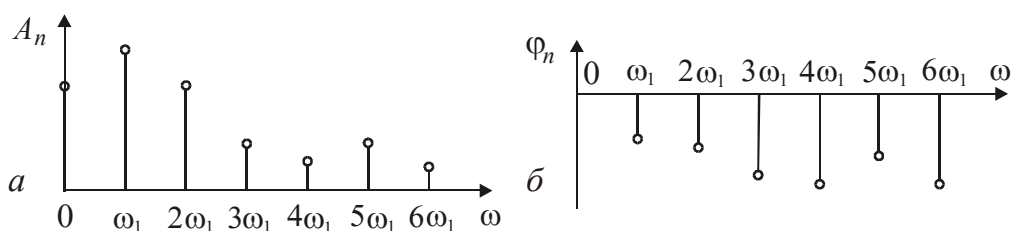
Рис. 1.1. Амплитудная и фазовая спектральные диаграммы
