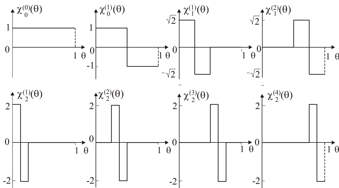
Рис.5.1. Графики первых восьми функций Хаара
