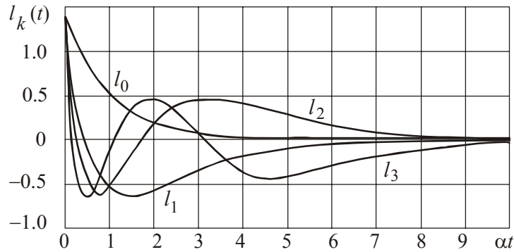
Рис. 3.1. Графики первых четырех функций Лагерра
