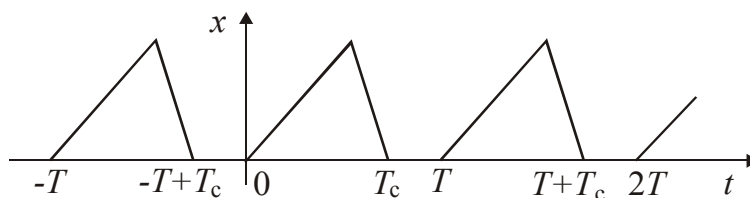
Рис. 1.2. Пример периодического сигнала
