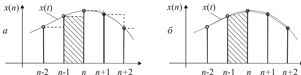
Рис. 8.1. Геометрическое представление интегрирования: a – по методу прямоугольников, b – по методу трапеций
