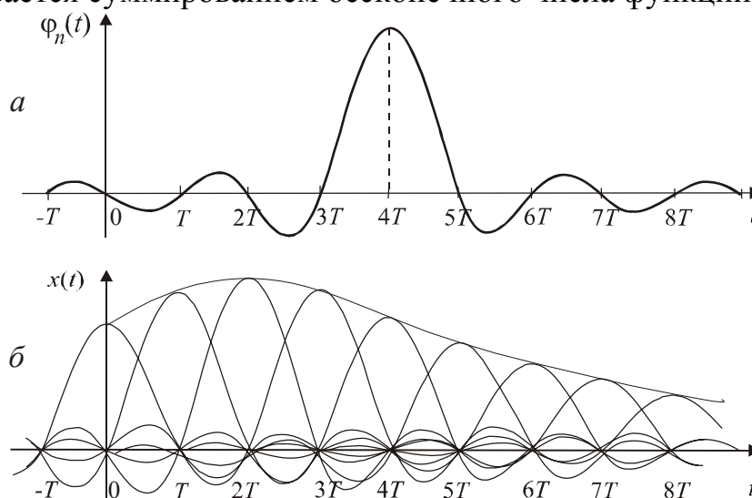
Рис. 7.1. Представление сигнала в виде ряда Котельникова: а – отсчетная функция; б – составляющие ряда
