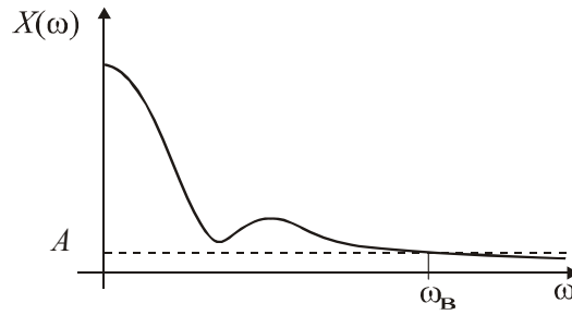
Рис. 7.2. Определение границы частотного интервала
