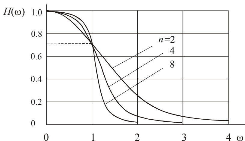
Рис. 6.1. АЧХ нормированных фильтров Баттерворта
