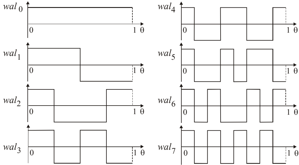
Рис. 4.2. Система Уолша, состоящая из N = 2^3 = 8 функций
