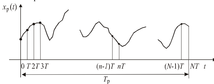
Рис. 12.1. Дискретизация реализации случайного процесса
