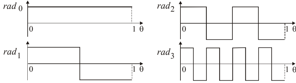
Рис. 4.1. Функции Радемахера
