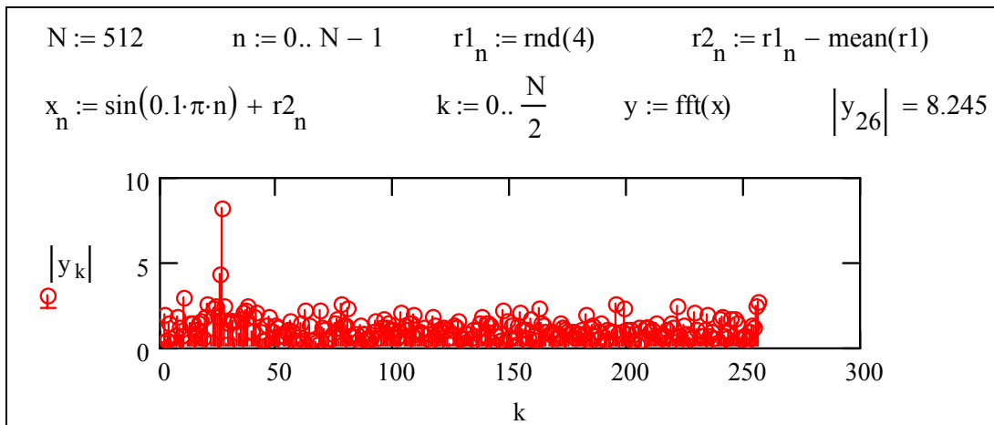
Рис. П.5. Пример использования БПФ
