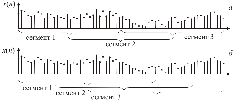
Рис. 14.1. Варианты перекрытия сегментов: а – с коэффициентом перекрытия D = 0.5 ; б – с коэффициентом перекрытия D = 0.75
