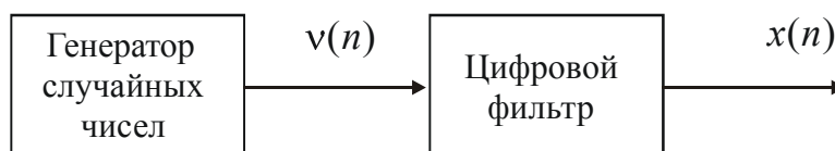
Рис. 12.2. Формирование последовательности случайных чисел
