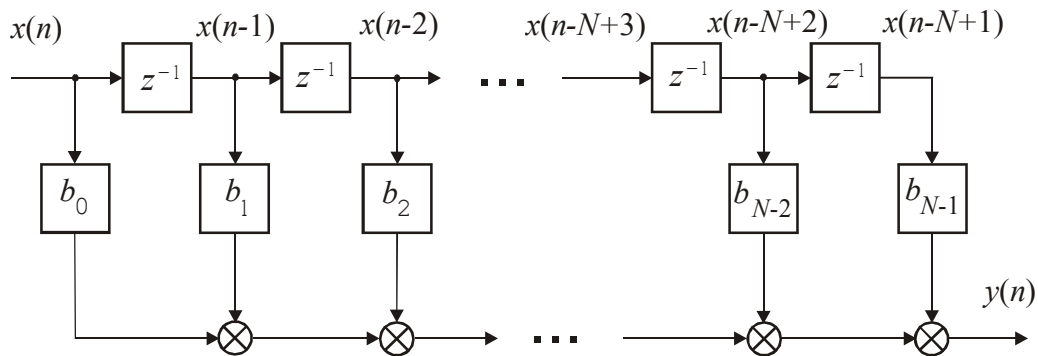
Рис. 11.1. Структурная схема нерекурсивного цифрового фильтра
