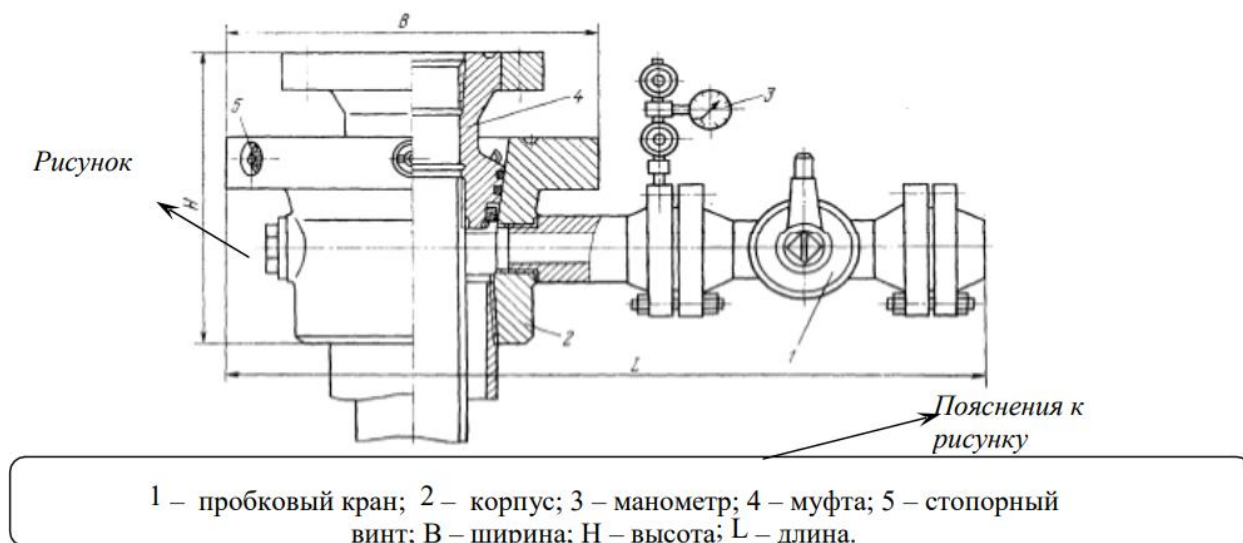
Рисунок 1.3 – Оборудование обвязки обсадных колонн типа ОКМ
