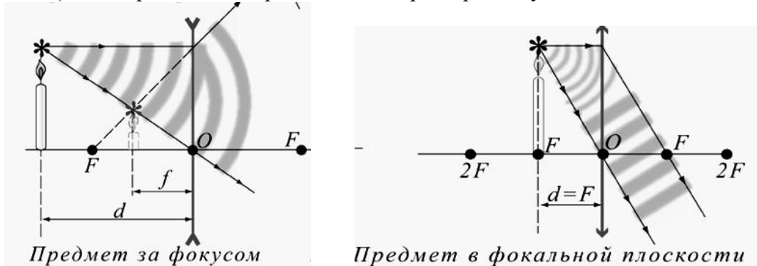
Рис. 4. Построение изображений в рассеивающей линзе.
