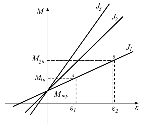
Рис. 24. Зависимость момента силы натяжения нити от углового ускорения.
