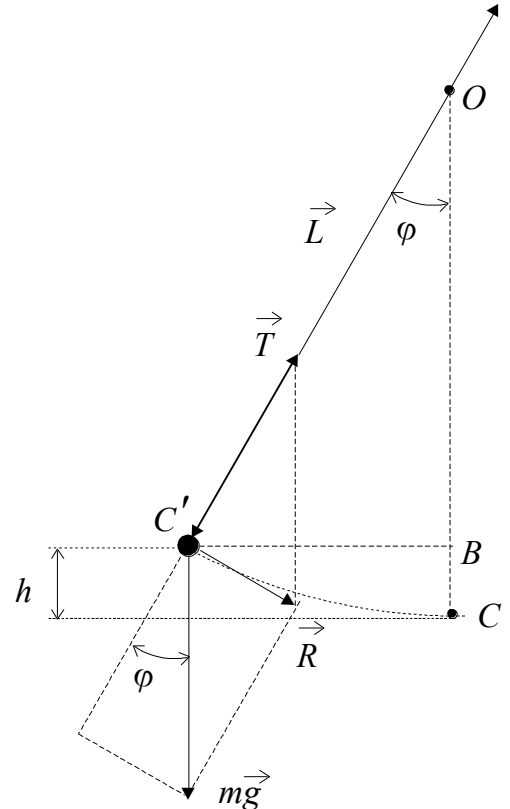
Рис. 1. Математический маятник
