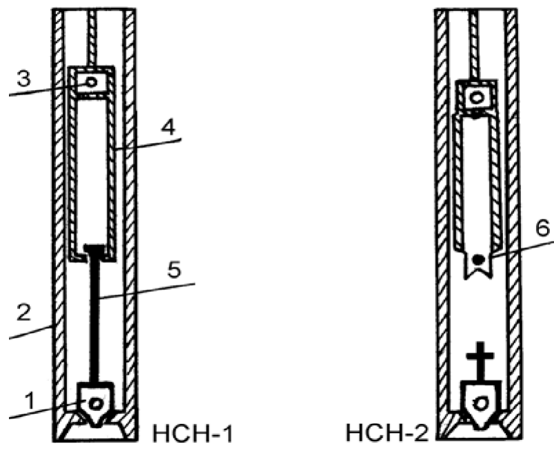
Рис. 15. Невставные скважинные насосы:
