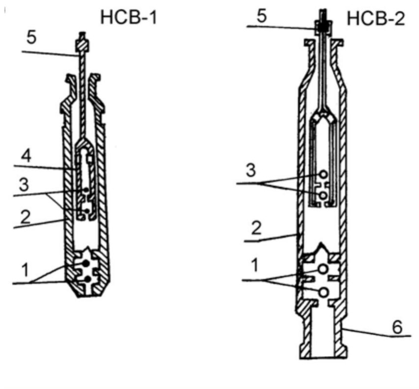
Рис. 14. Насосы скважинные вставные
