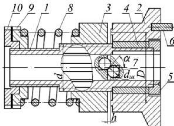
Рисунок 9.2 – Пружинно-шариковая муфта
