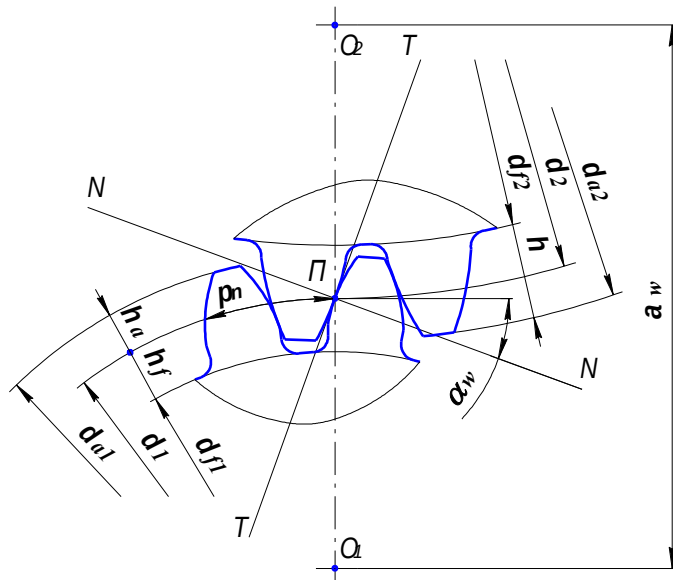
Рис. 3.1 – Зубчатое зацепление
