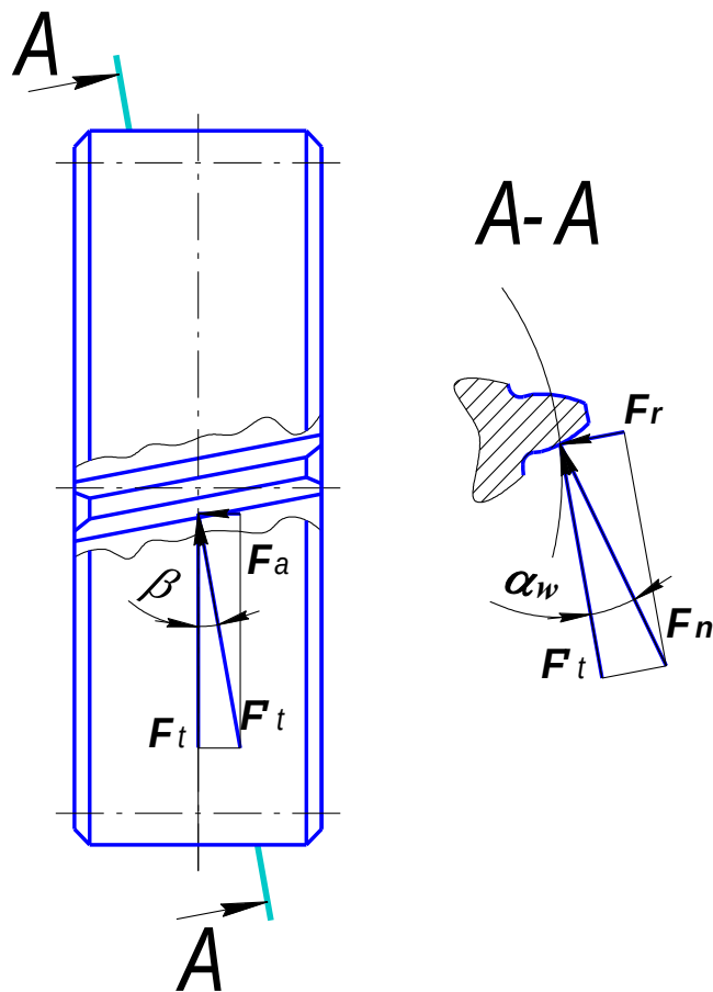
Рисунок 2.1. – Силы в прямозубом зацеплении Силы в косозубом зацеплении
