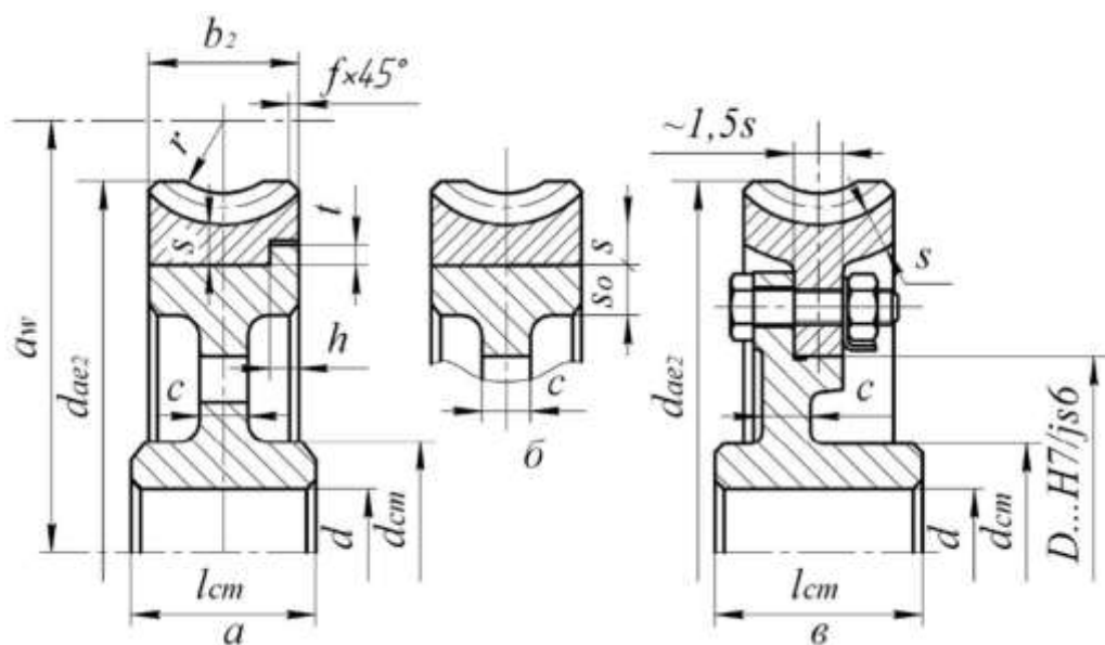
Рисунок 4 – Конструкции червячных зубчатых колес
