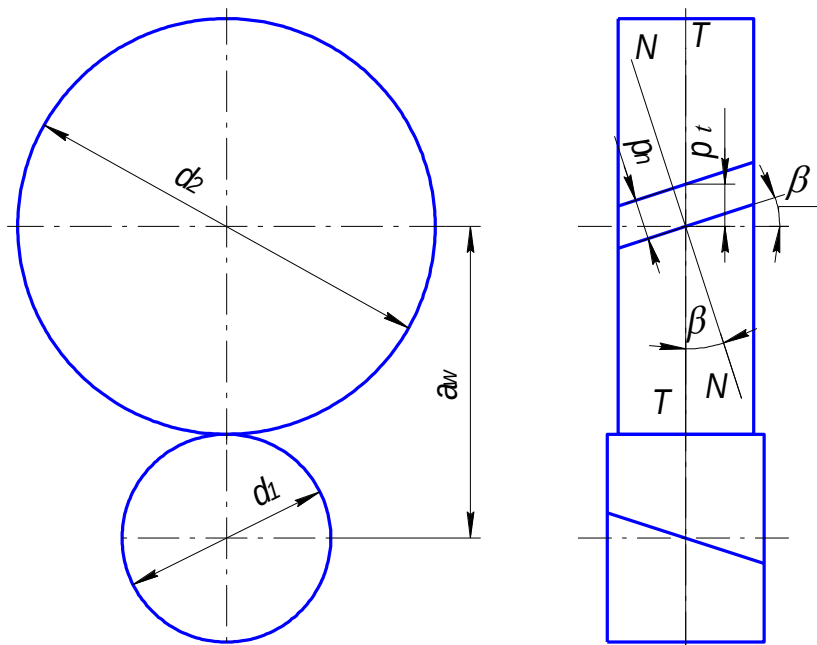
Рис. 3.2 – Косозубая передача
