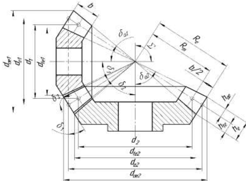
Рисунок 3 –Схема конического зацепления Делительные диаметры зубчатых колес
