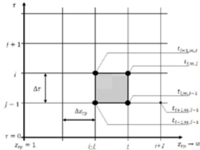
Рисунок 4 – Конечно-разностная схема по координатам z_{\text{гп}} - \tau , для расчетного m
