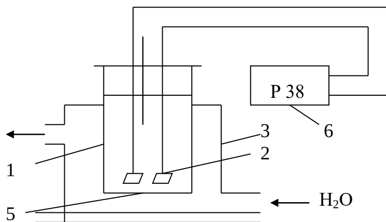
Рис. 9.11. 1- ячейка для измерений электропроводности с платинированными электродами (2); 3- терморегулируемый блок , 4- термопара, 5- магнитная мешалка, 6- мост переменного тока Р-38 или Р-5021.
