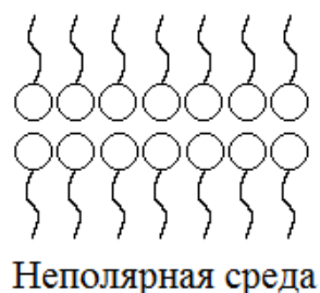
Рис. 9.8. «Обратная» мицелла Мак-Бена
