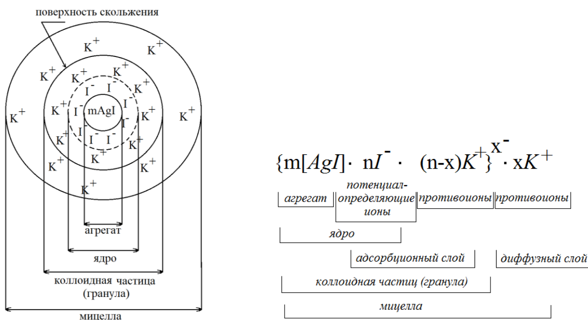
Рис. 1.1. Схема строения мицеллы золь иодида серебра с отрицательно заряженными частицами и её формула
