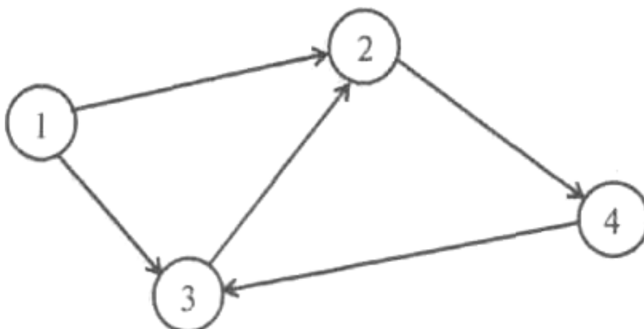
Рисунок 4.1 – Пример орграфа с контуром
