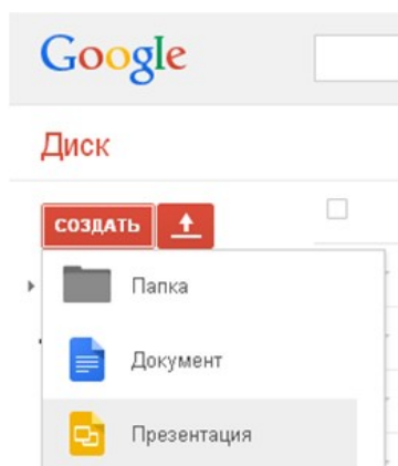
Рисунок 9.14 – Создание презентации
