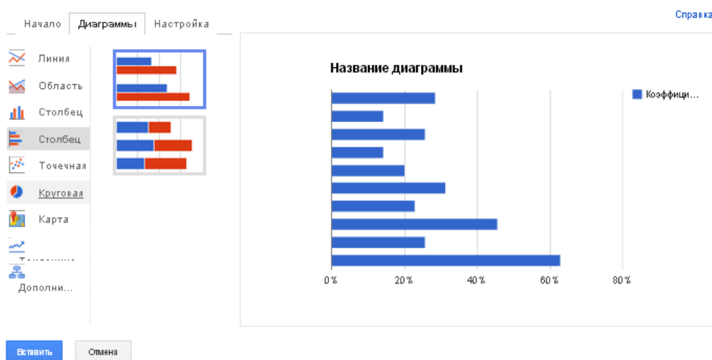
Рисунок 9.29 - Типы диаграмм
