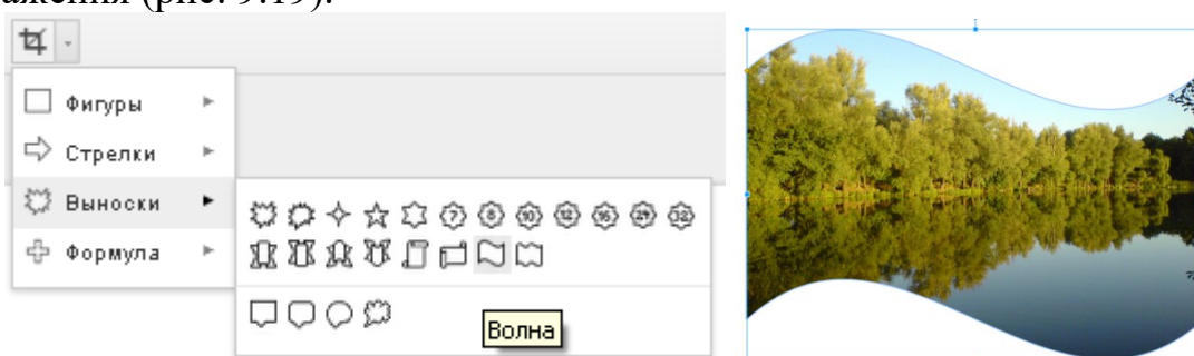
Рисунок 9.19 – Операция кадрирования
