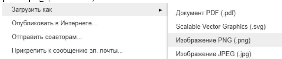
Рисунок 10.5 – Выбор формата
