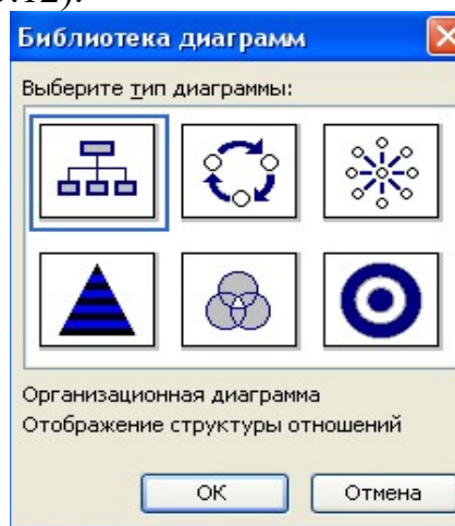
Рисунок 5.12. – Библиотека диаграмм
