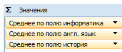
Рисунок 3.12.
