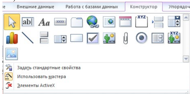
Рисунок 4.18. - Элементы управления
