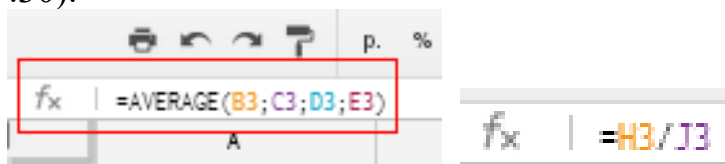
Рисунок 9.30 – Ввод формул
