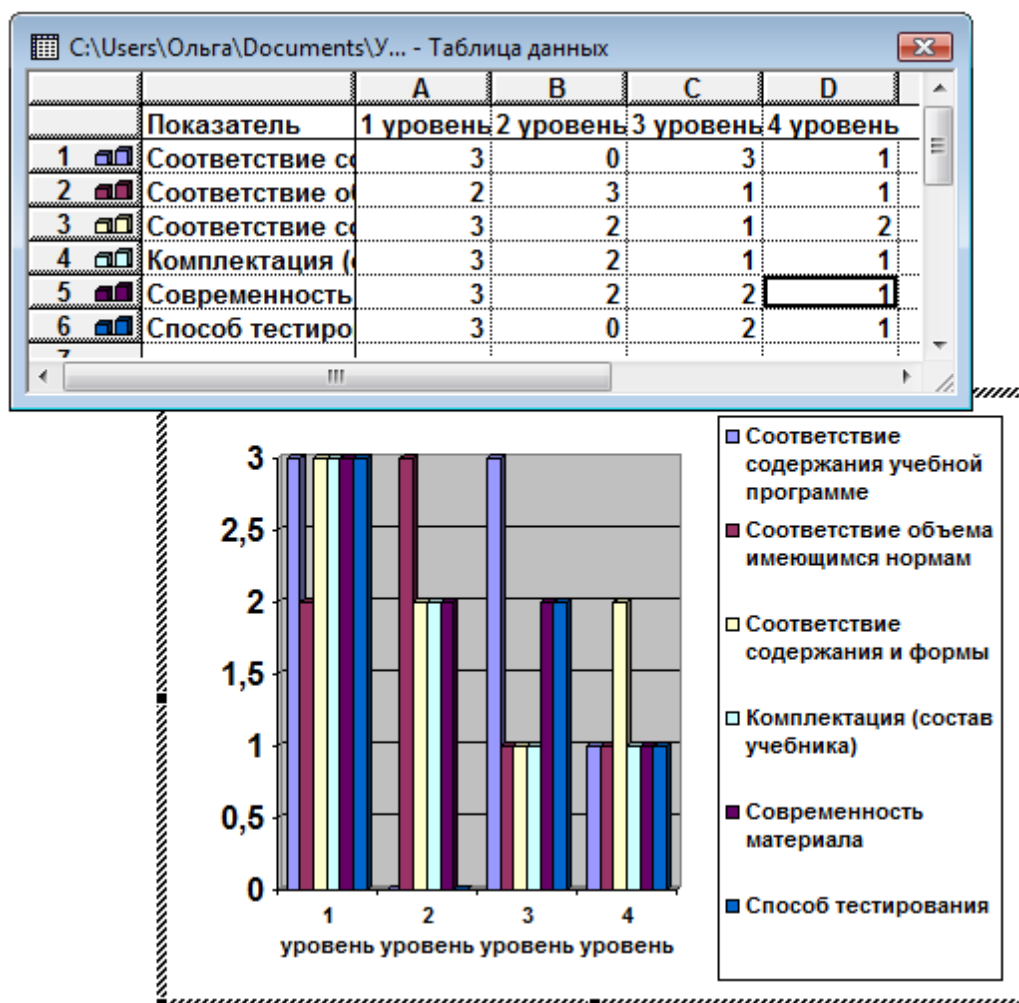
Рисунок 2.4. Диаграмма
