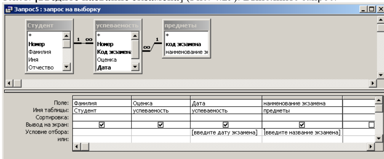
Рисунок 4.29. - Запрос параметром
