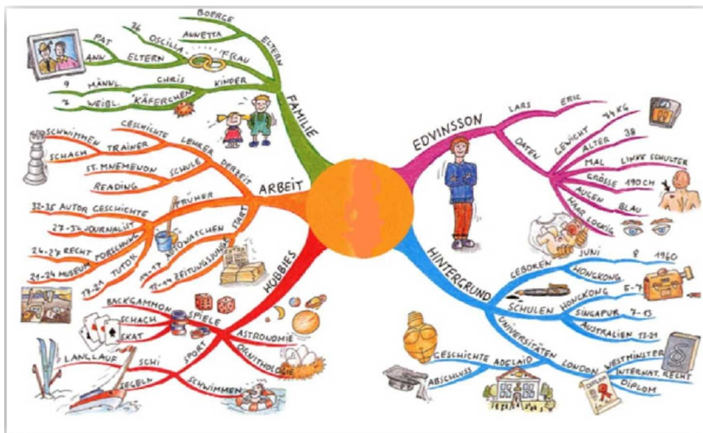
Рисунок 10.6 – Примеры интеллект-карт
