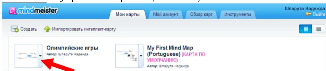
Рисунок 10.9 – Окно программы
