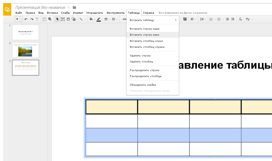
Рисунок 9.21 – Редактирование таблицы
