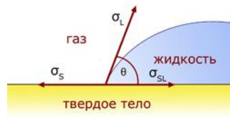
Рисунок 2.1. Геометрия капли, лежащей на твердой поверхности
