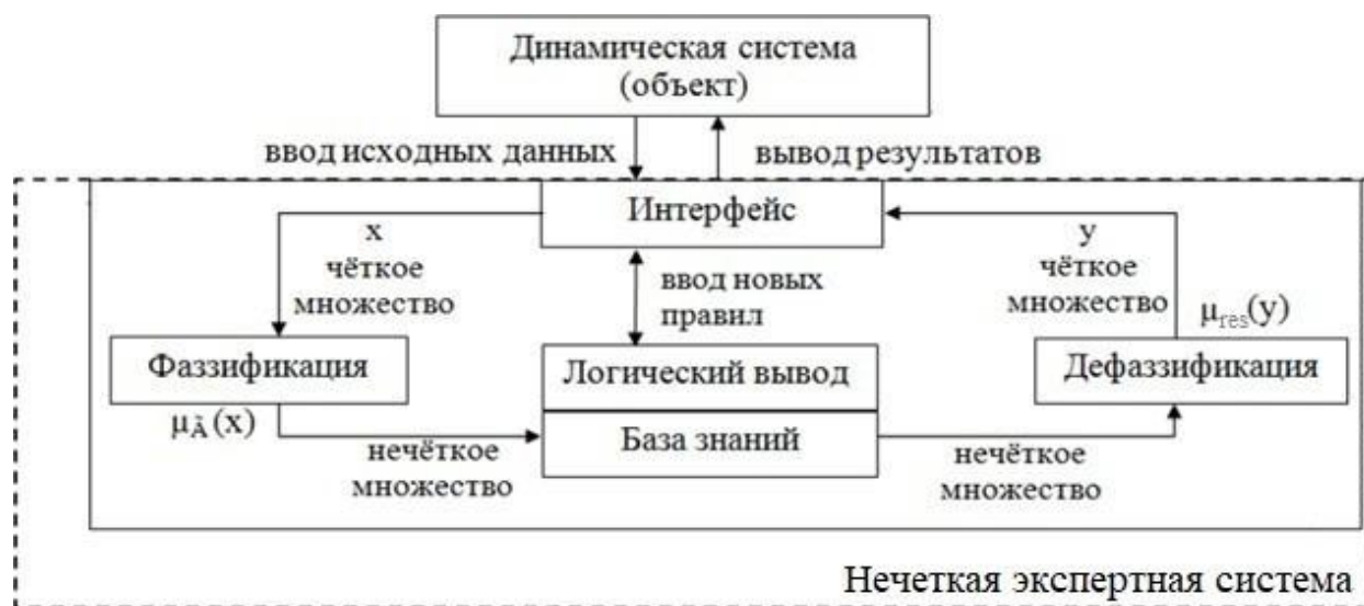
Рис. 1.2. Структура НЭС
