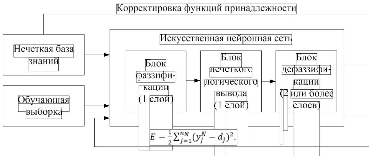
Рис. 4.1. Общая структура гибридной нейро-нечеткой системы
