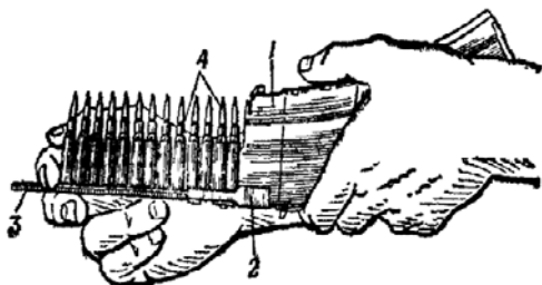
Рис. 63. Снаряжение магазина патронами из обоймы:
