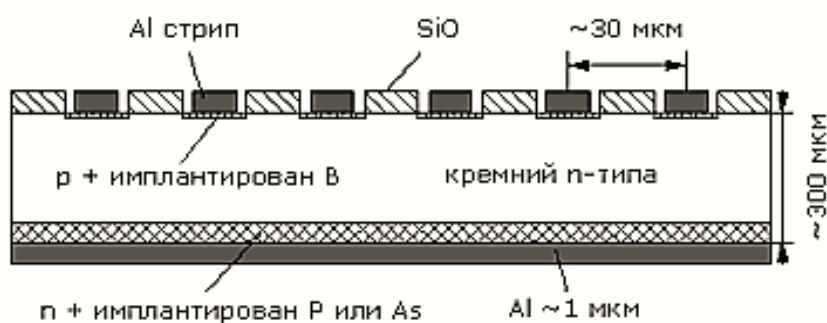
Рисунок 2.5 – Устройство кремниевого микроstriпового детектора
