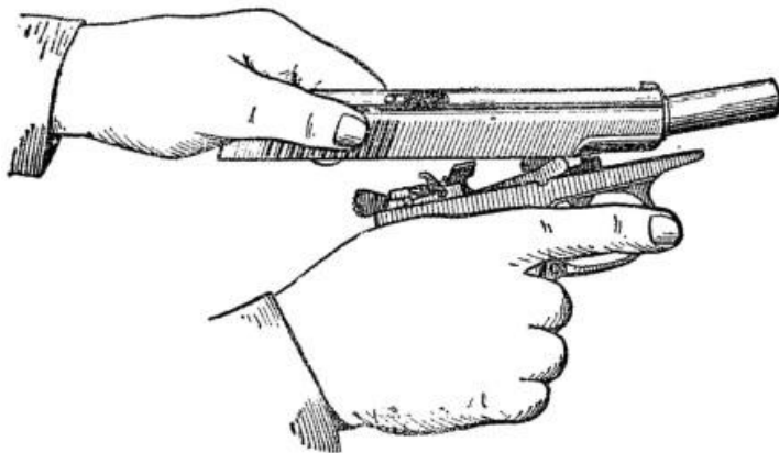
Рис. 7. Присоединение затвора к рамке
