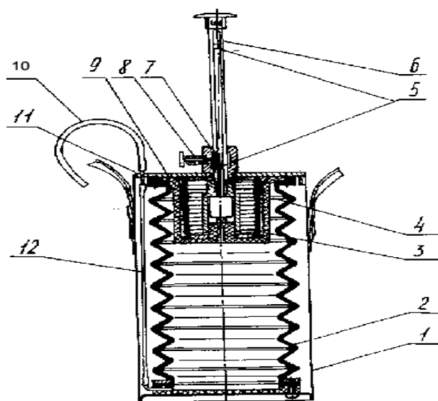
Рис. 12. Газоанализатор УГ-2
