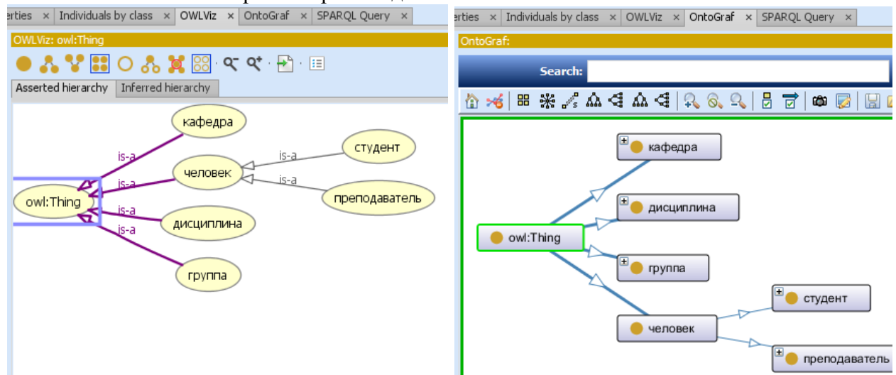
а) OWLViz
