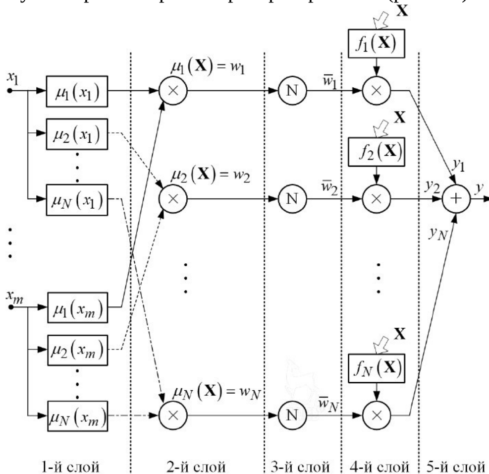
Рис. 4.2. Структура ANFIS-сети
