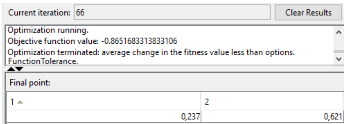
Рис. 5.12. Результаты поиска минимума функции
