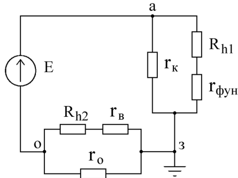
Рисунок 10 – Расчетная эквивалентная схема
