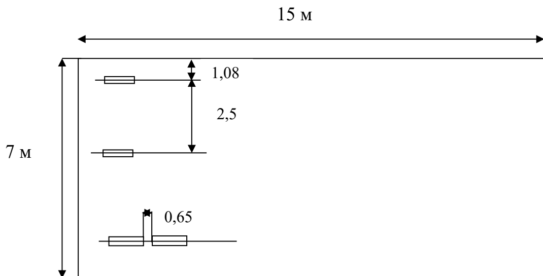
Рисунок 5 – Размещение светильников в помещении
