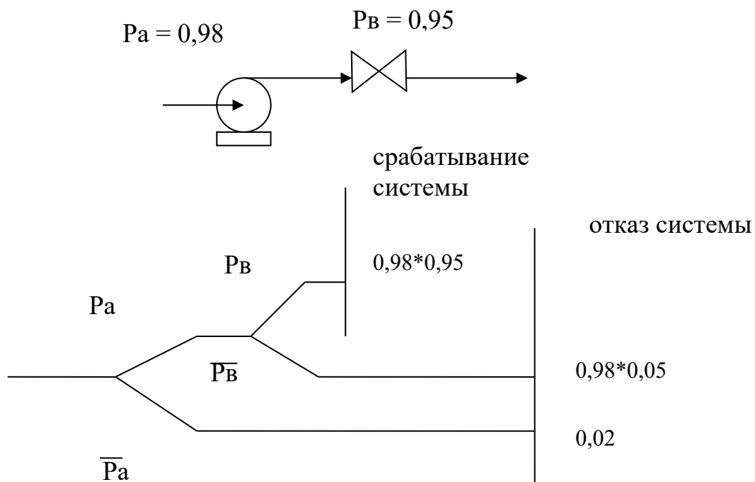
Рисунок 1 – Расчетная схема
