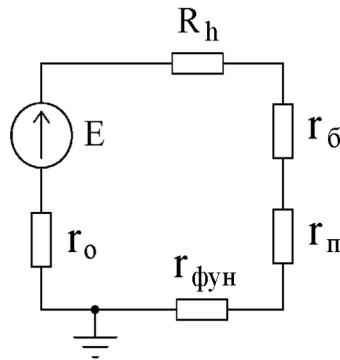
Рисунок 8 – Расчетная эквивалентная схема
