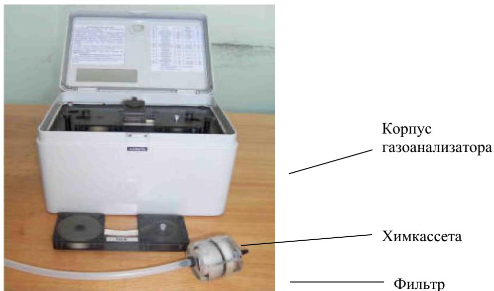
Рисунок 3.2 – Общий вид газоанализатора ГАНК-4
