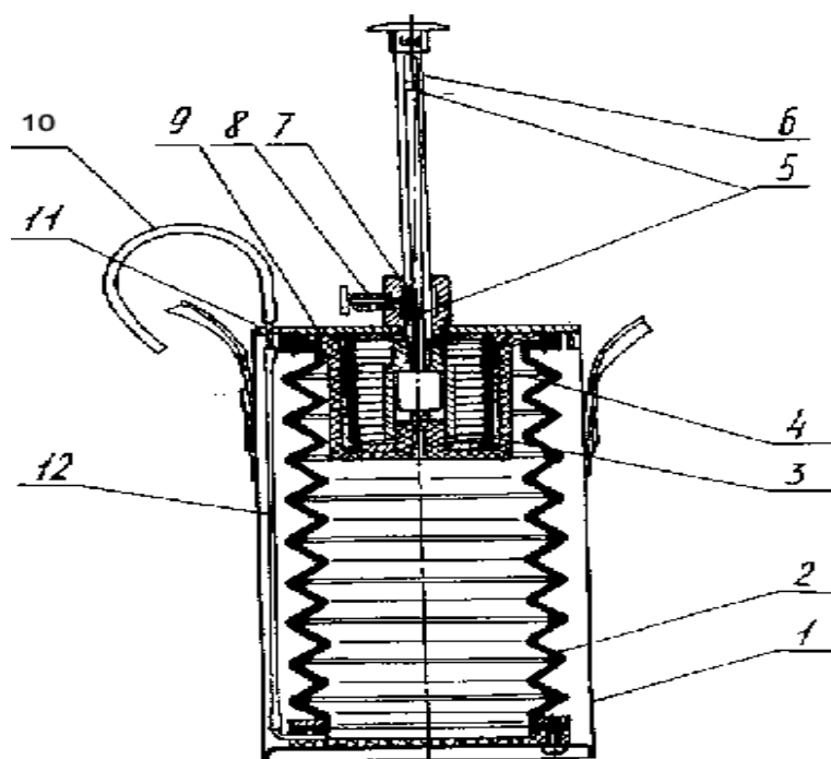
Рис. 12. Газоанализатор УГ-2
