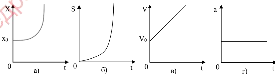
Рисунок 2. График зависимости а) x = f(t) ; б) S = f(t) ; в) V = f(t) ; г) a = f(t)
