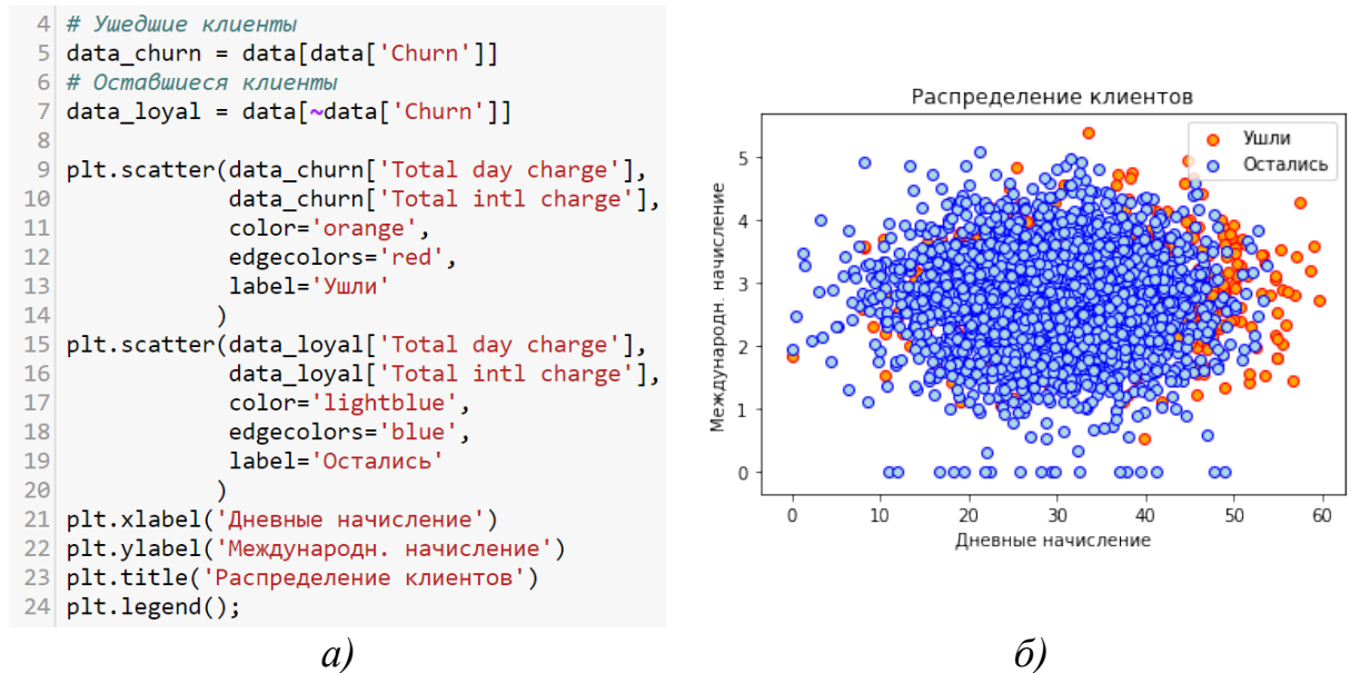
Рисунок 2.17 – Построение отдельных подмножеств с легендой; а) исходный код; б) полученный график
