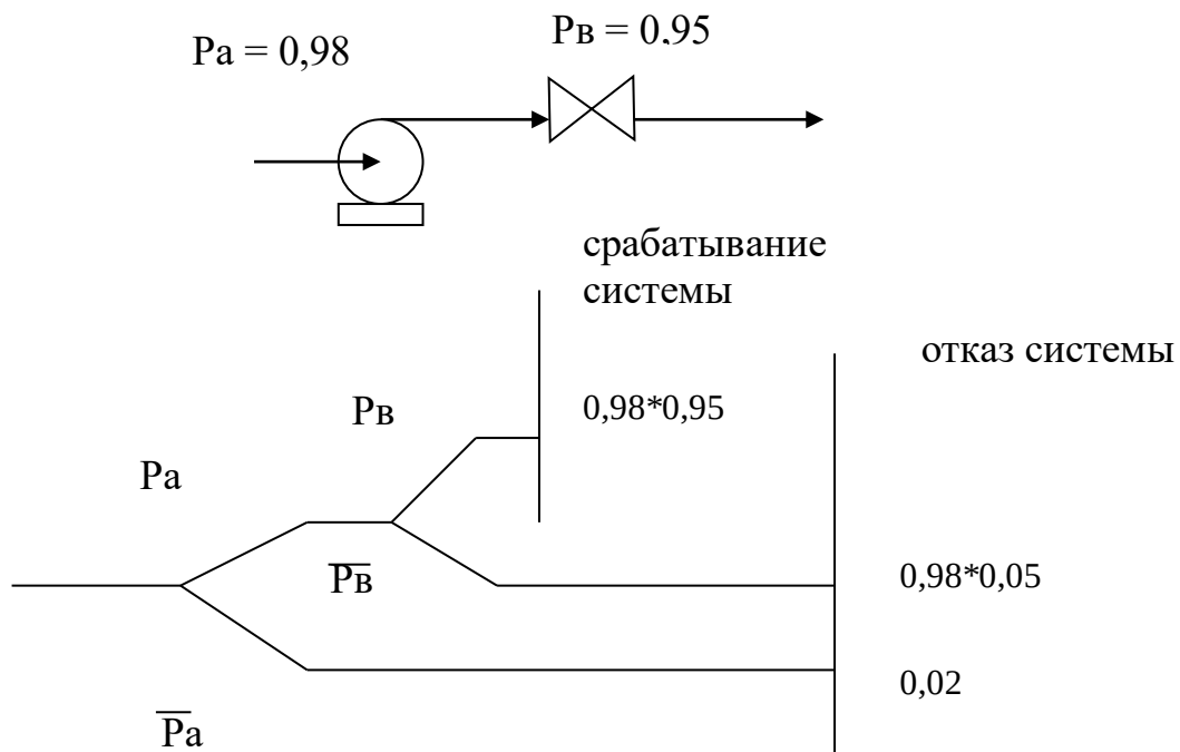
Рисунок 6.1 – Расчетная схема
