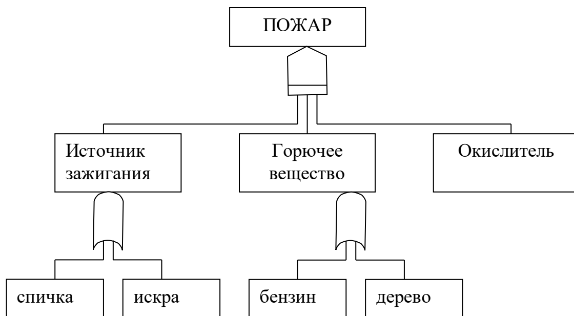
Рисунок 2.2 – Дерево событий
