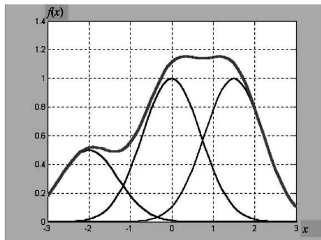
Рис. 4. Функция f(x)
