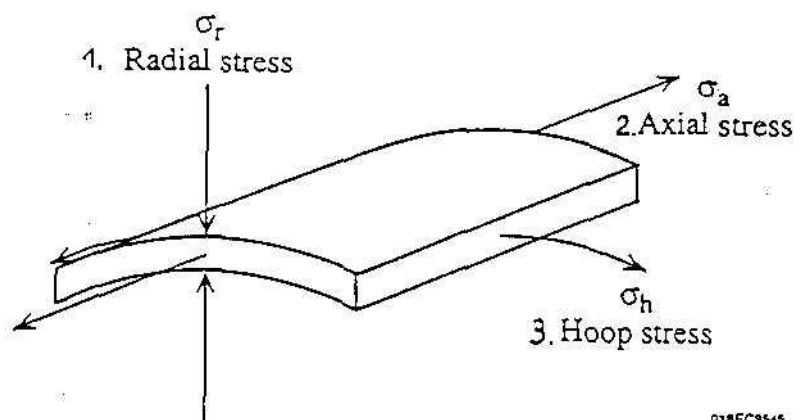
Рис. 3.1. Три основных вида напряжений, возникающих в гибких НКТ:
