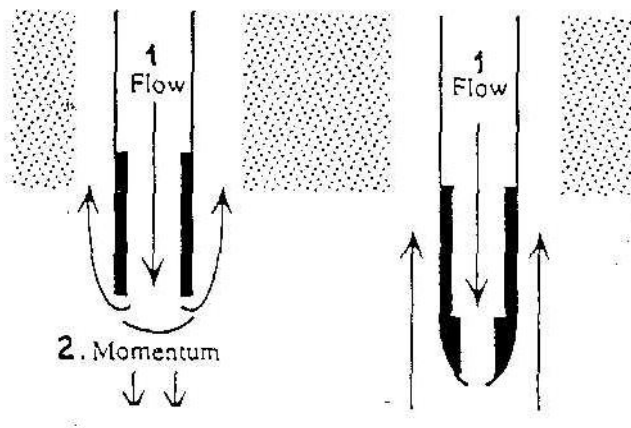
Рис. 1.4. Силы, возникающие при циркуляции жидкости:
