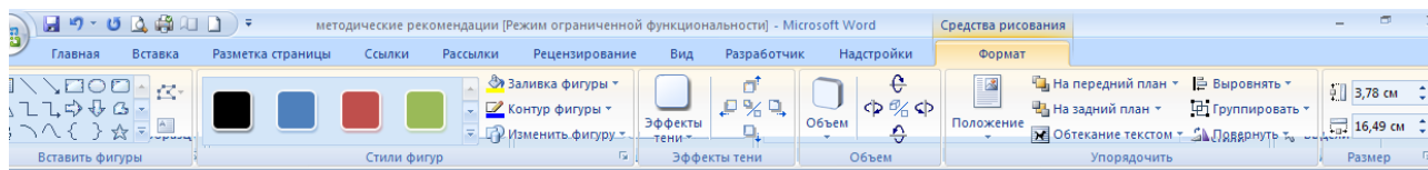
Рис.1. Средства рисования
