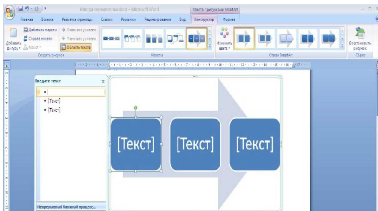
Рис. 5. Объекты SmartArt
