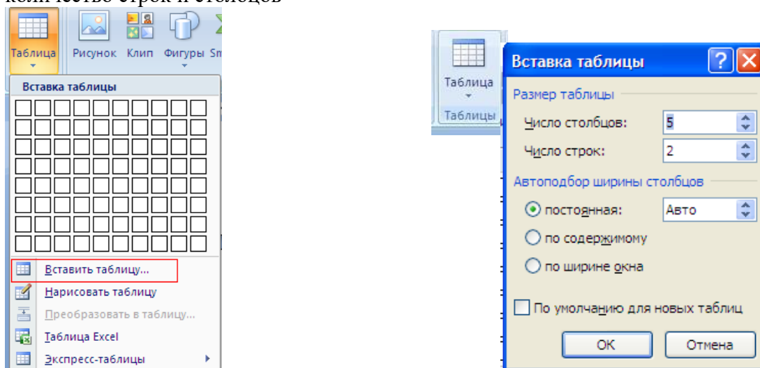
Рис.1. Создание таблицы
