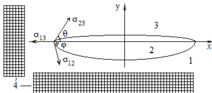
Рисунок 2.2. Схема опыта и условие равновесия трех фаз (1 – воды, 2 – твердый стеарин, 3 – воздух, 4 – масштабные линейки)
