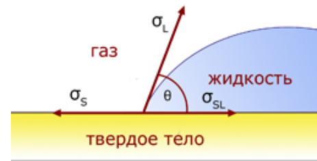
Рисунок 2.1. Геометрия капли, лежащей на твердой поверхности
