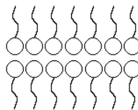
Неполярная среда
