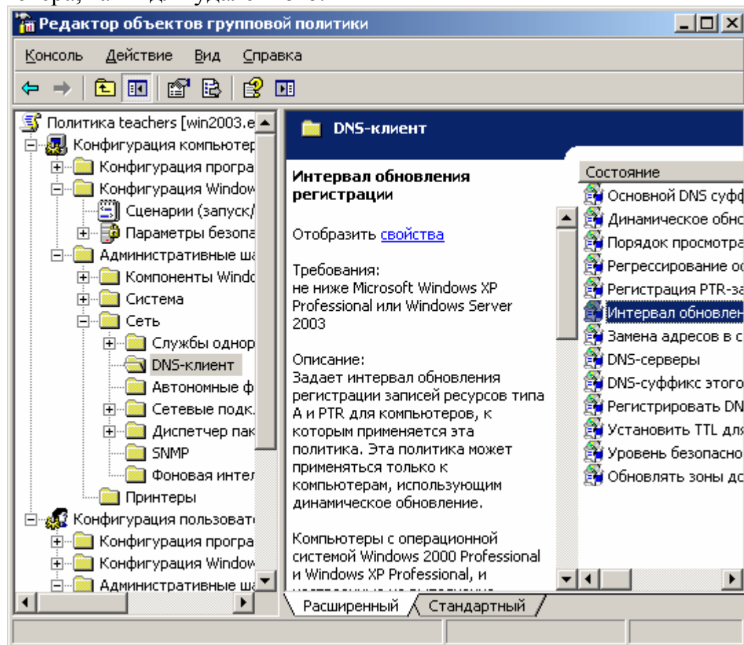
Рисунок 1. Редактор объектов групповой политики.
