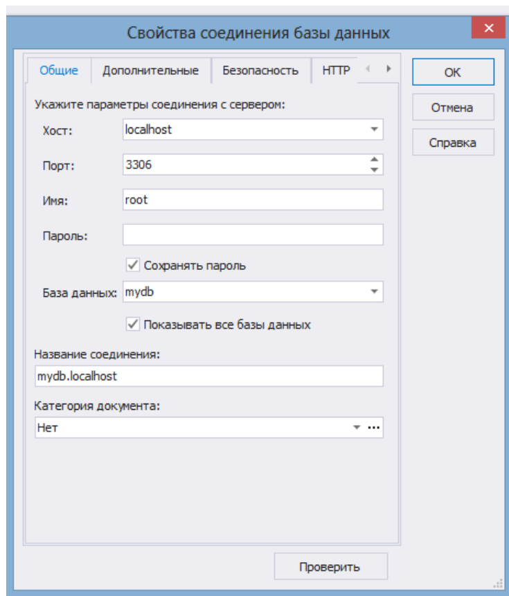
Рисунок 16.1 – Этап 1
