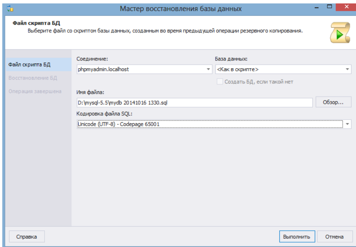
Рисунок 16.7 – Этап 8 165
