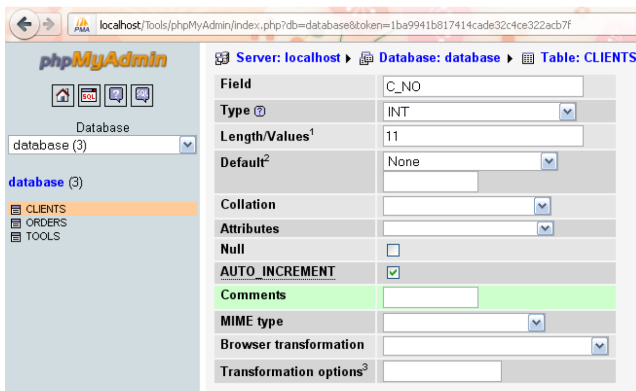
Рисунок 6.1 – Добавление AUTO_INCREMENT
