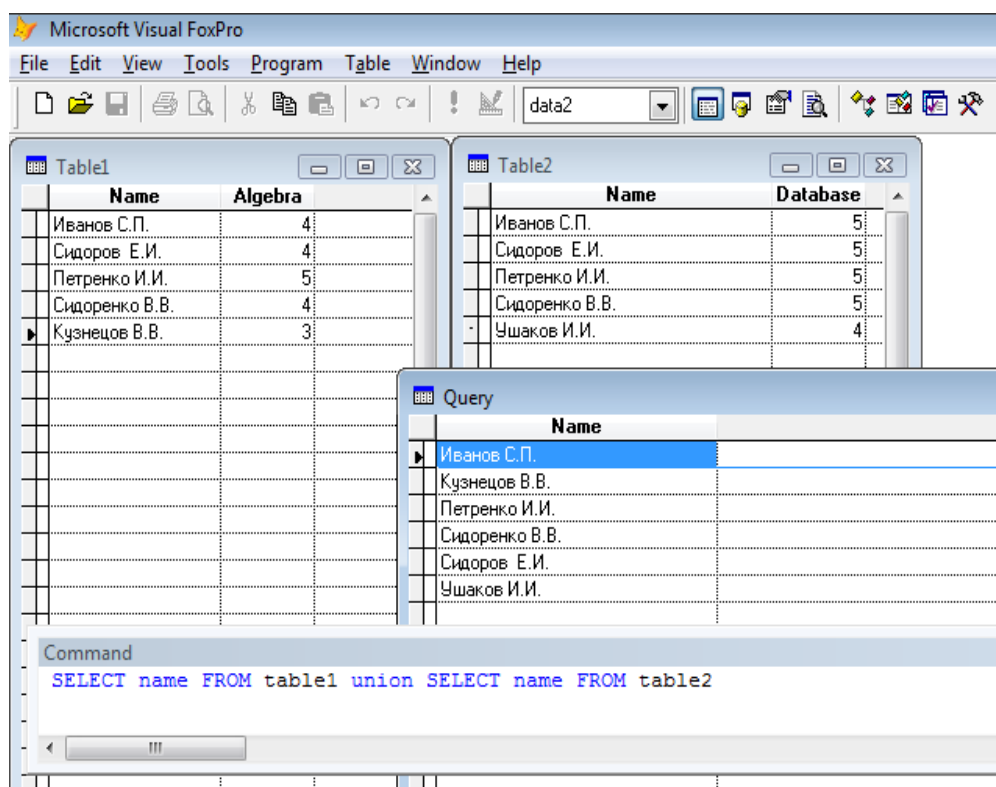
Рисунок 13.1 – Объединение таблиц
