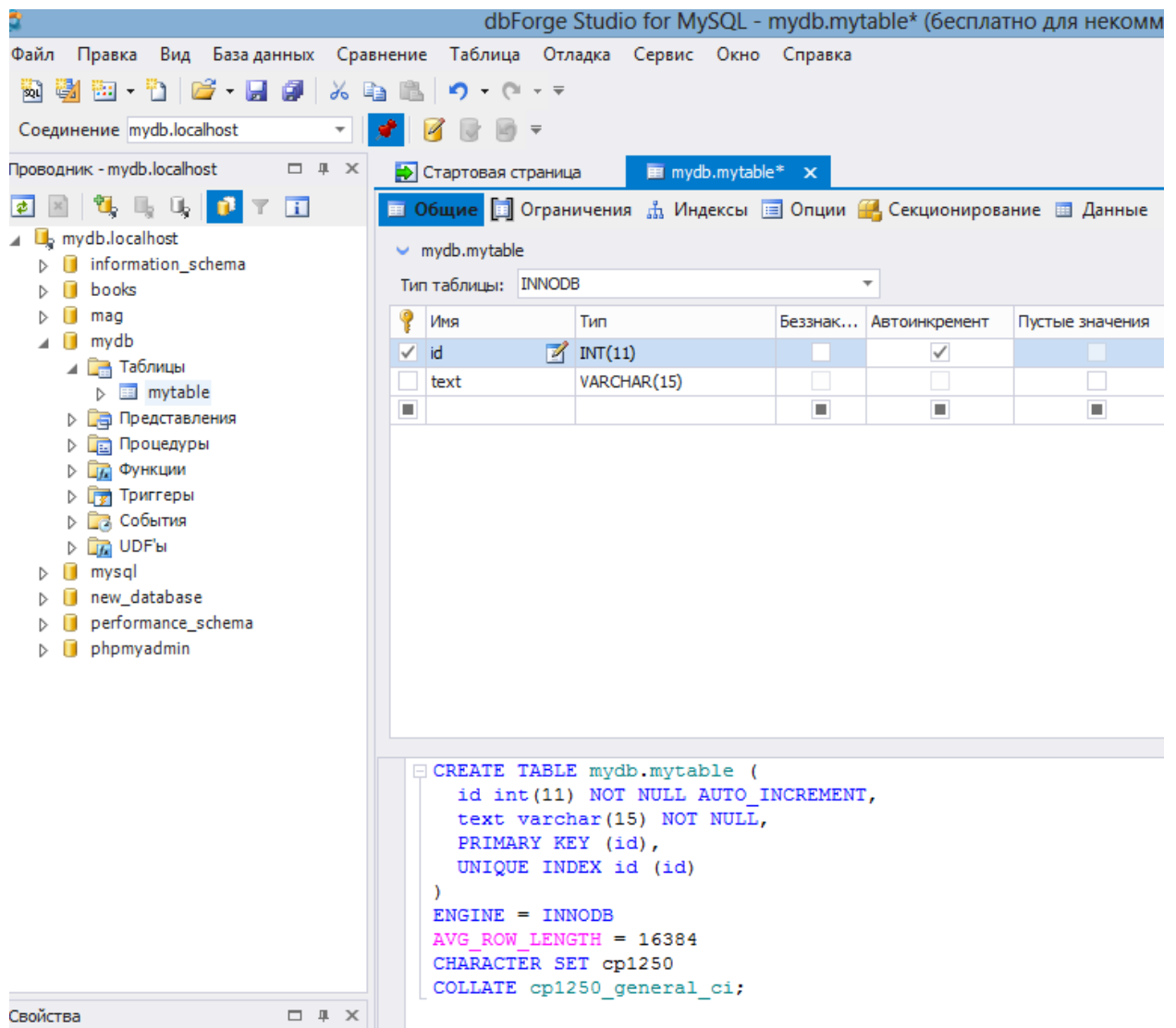
Рисунок 16.2 – Этап 3
