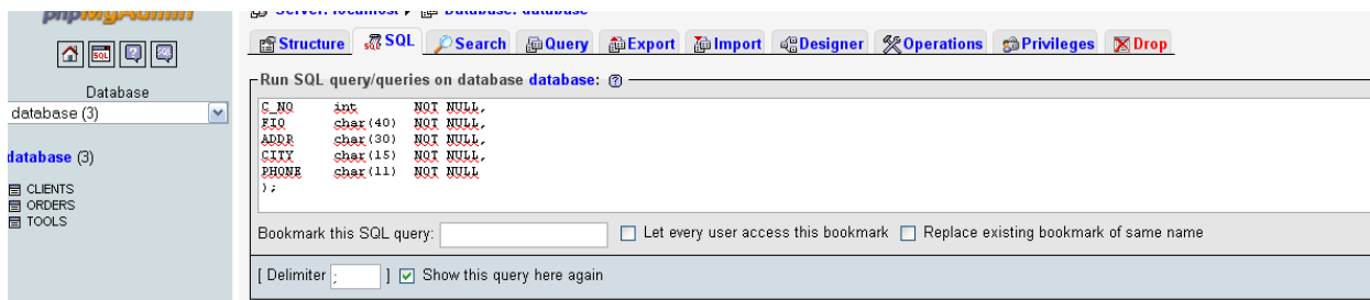
Рисунок 5.1 – Создание БД
