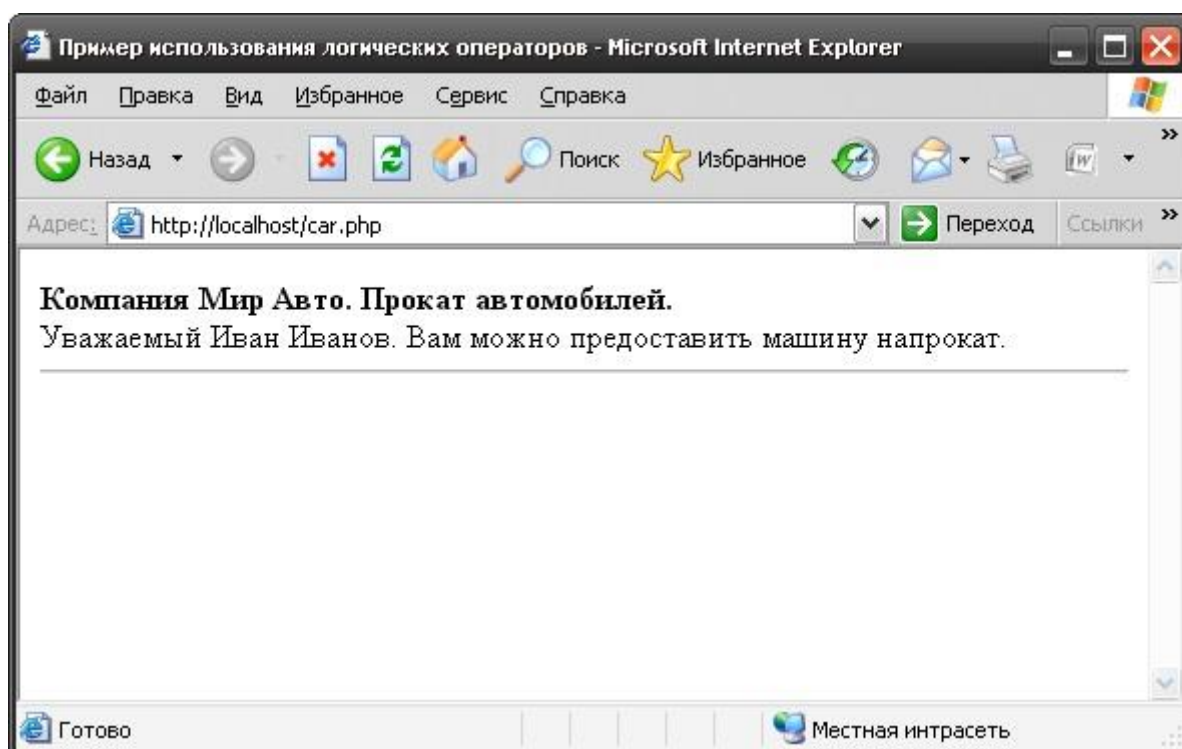
Рисунок 13.6 – Результат проверки
