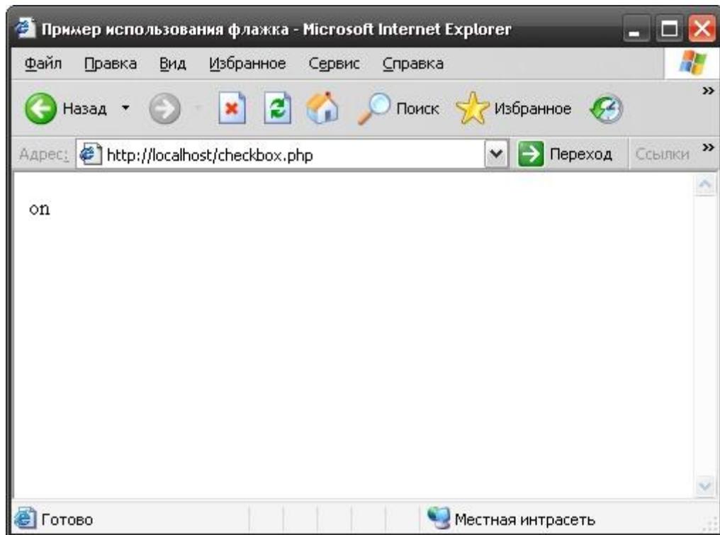
Рисунок 11.7 – Результат проверки
