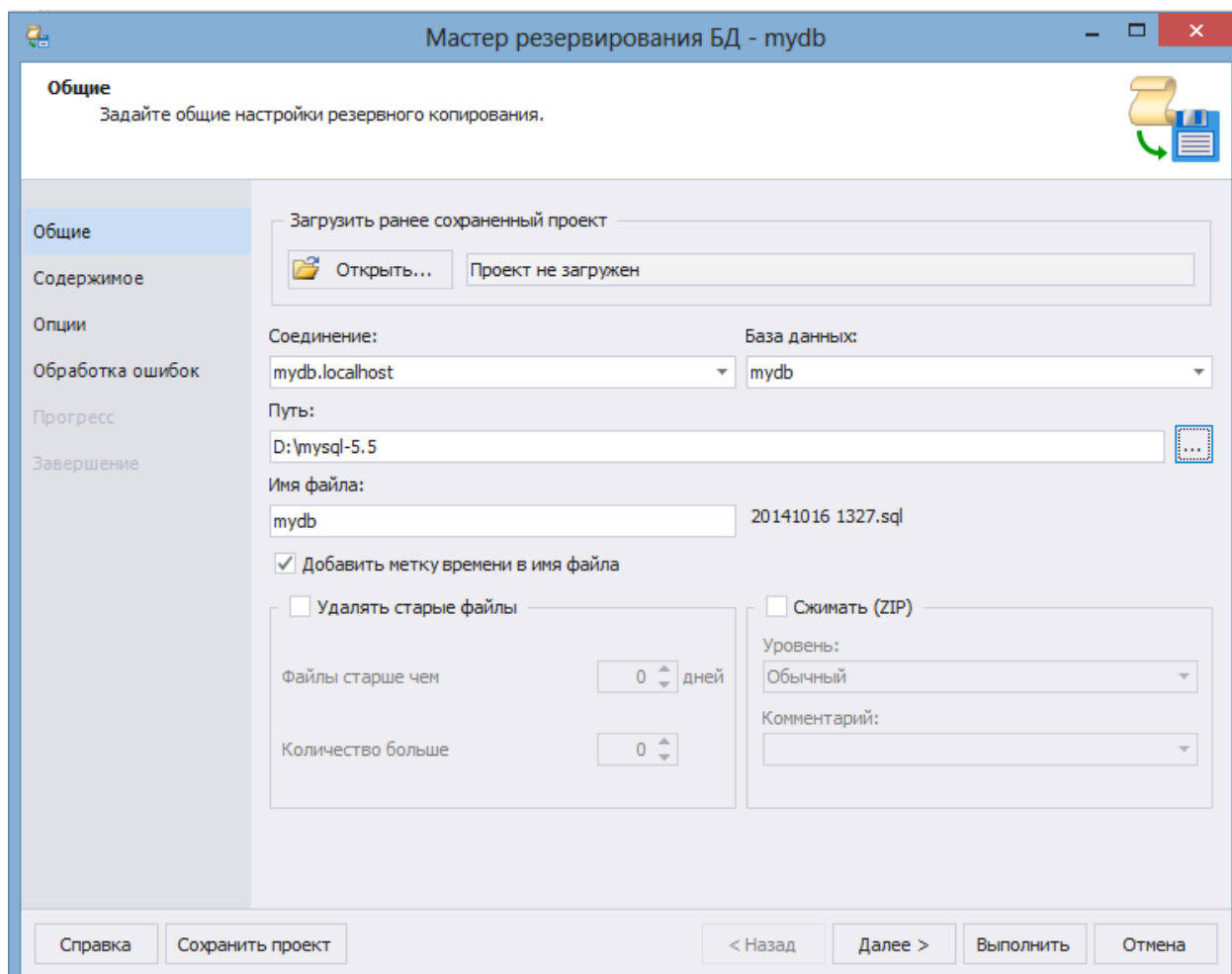
Рисунок 16.3 – Этап 4
