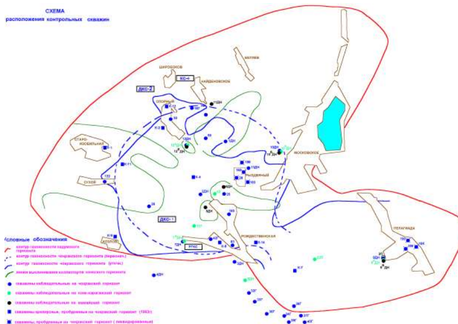
Рисунок 3. Схема расположения контрольных и наблюдательных скважин в системе контроля за герметичностью СС ПХГ
