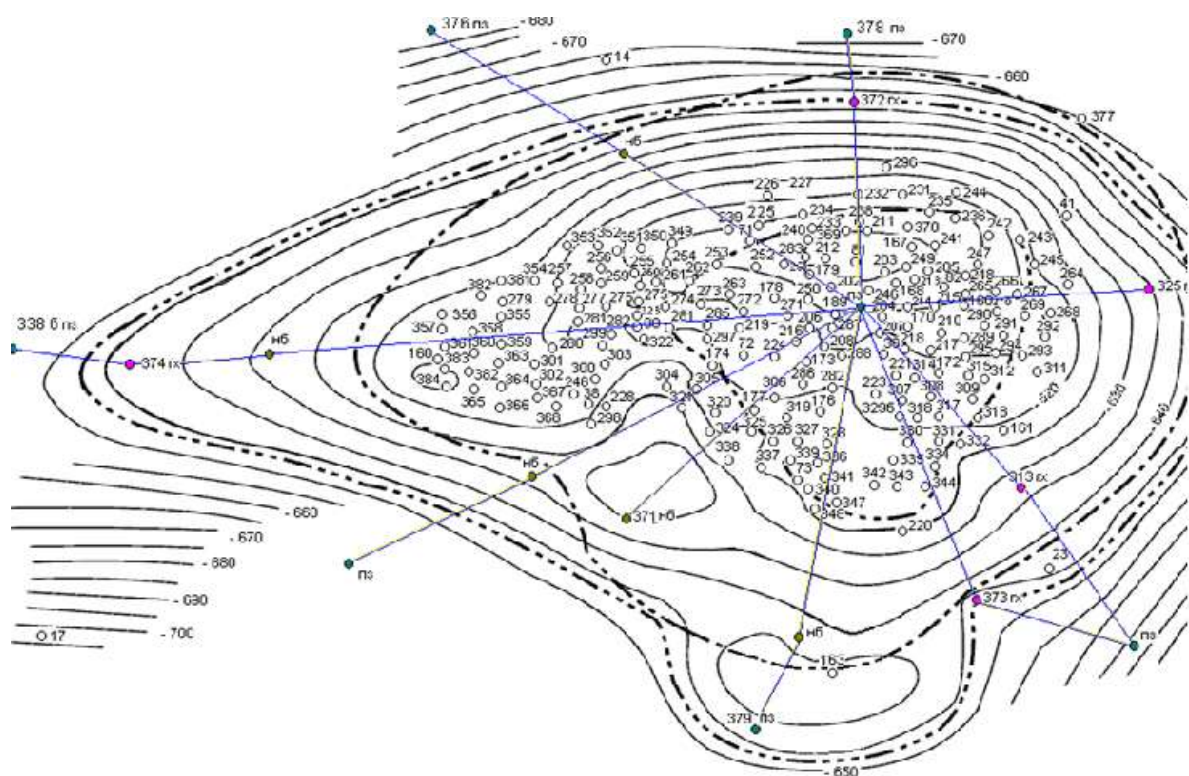
Рисунок 2. Схема расположения контрольных и наблюдательных скважин в горизонте зелёная свита СС ПХГ
