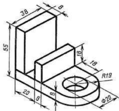
Кронштейн
