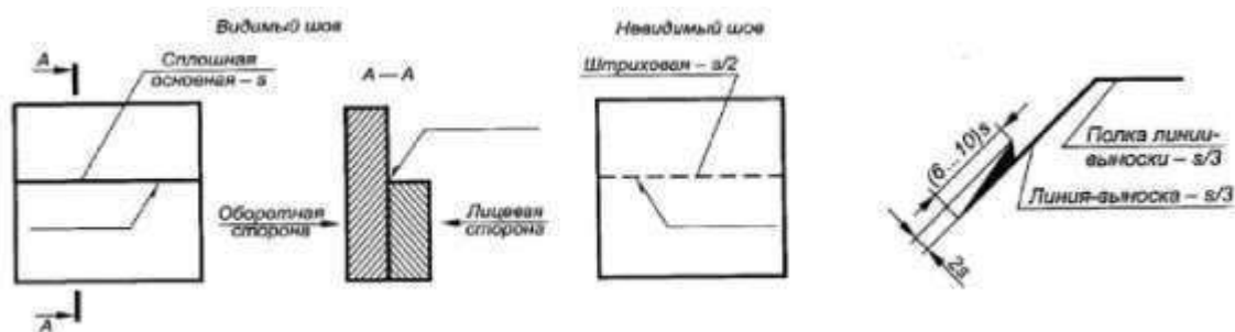
Рисунок 7.2–Изображение швов
