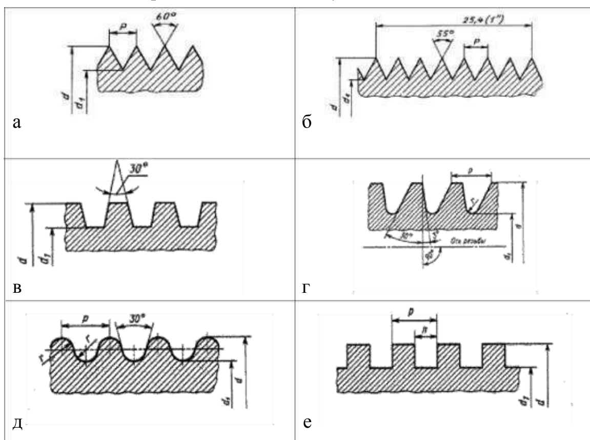
Рисунок 3.2. – Типы резьбы
