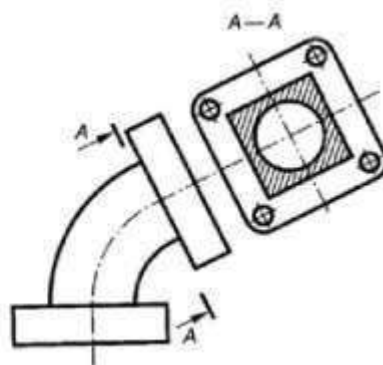
Рисунок 1.5 – Наклонный разрез
