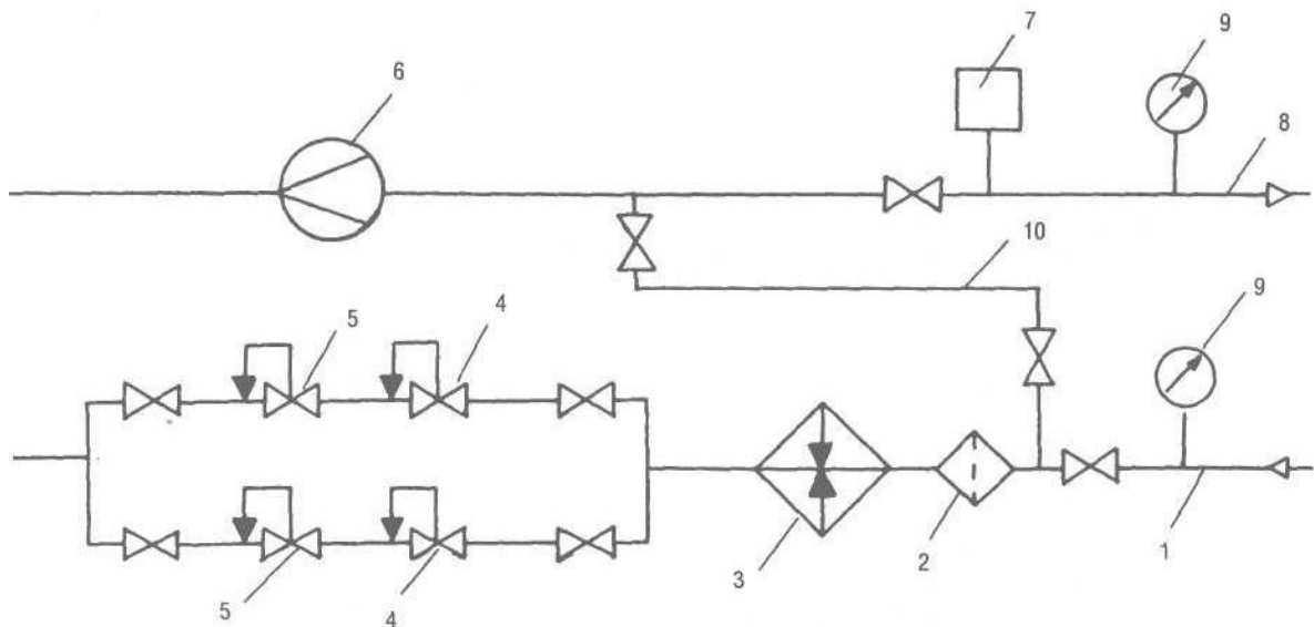
Рис. 26 – Принципиальная схема ГРС: 1 – входной трубопровод; 2 – фильтр; 3 – подогреватель газа; 4 – контрольный клапан; 5 – регулятор давления типа «послесебя»; 6 – расходомер газа; 7 – одоризатор; 8 – выходной трубопровод; 9 – манометр; 10 – байпас
