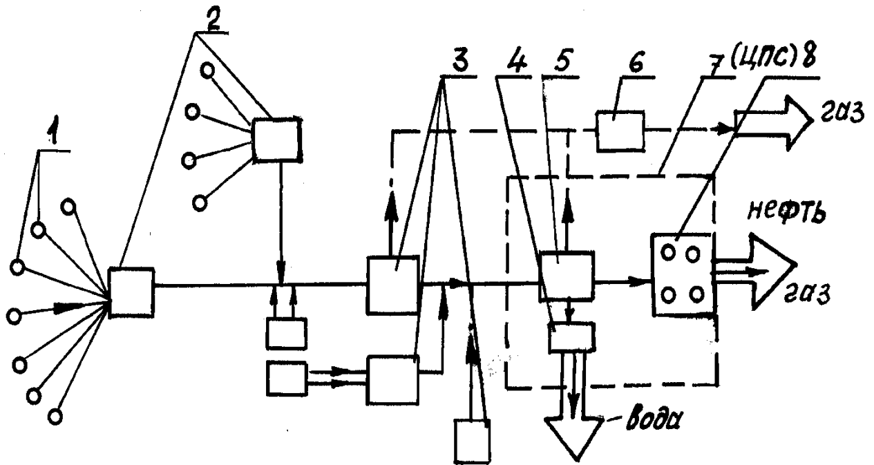
Рисунок 17 – Схема сбора и подготовки продукции скважин на нефтяном промысле: 1–нефтяная скважина; 2–автоматизированные групповые замерные установки (АГЗУ); 3– дожимная насосная станция (ДНС); 4–установка очистки пластовой воды; 5– установка подготовки нефти; 6–газокomppressorная станция; 7–центральный пункт сбора нефти, газа и воды; 8 –резервуарный парк
