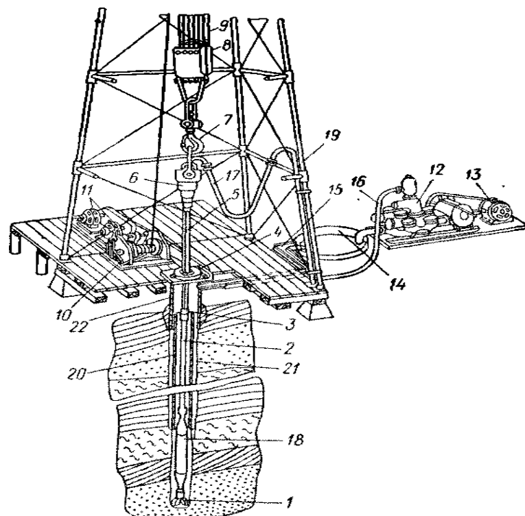
Рисунок 3 – Схема установки для бурения глубоких скважин роторными турбинными способами:
