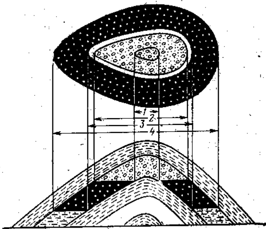
Рис.2.Сводоваягазонефтянаязалежь:1-внутреннийконтургазоносности;2-внешнийконтургазоносности;3-внутреннийконтурнефтеносности;4-внешний контур нефтеносности.
