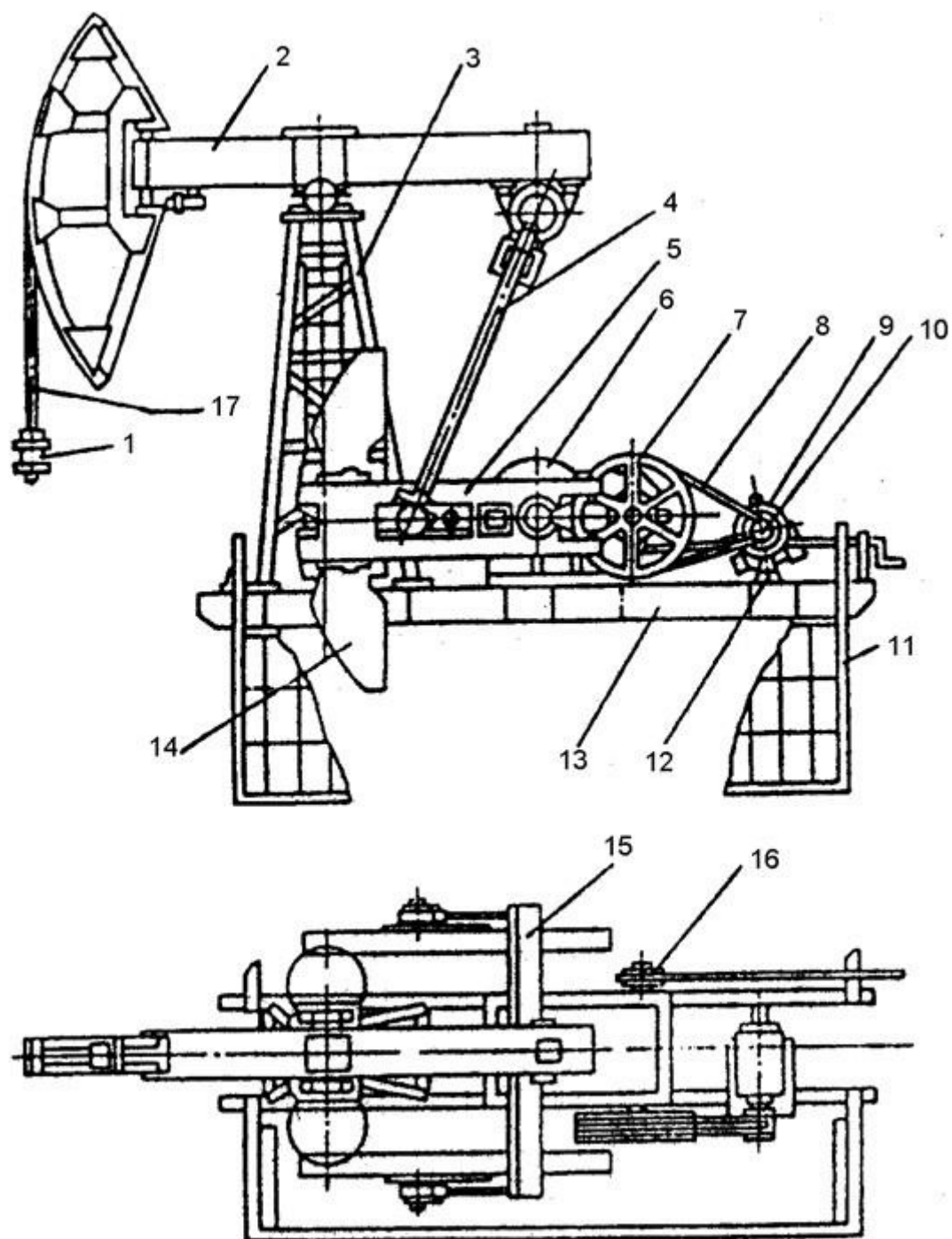
Рис.16. Станок-качалка типа СКД:
