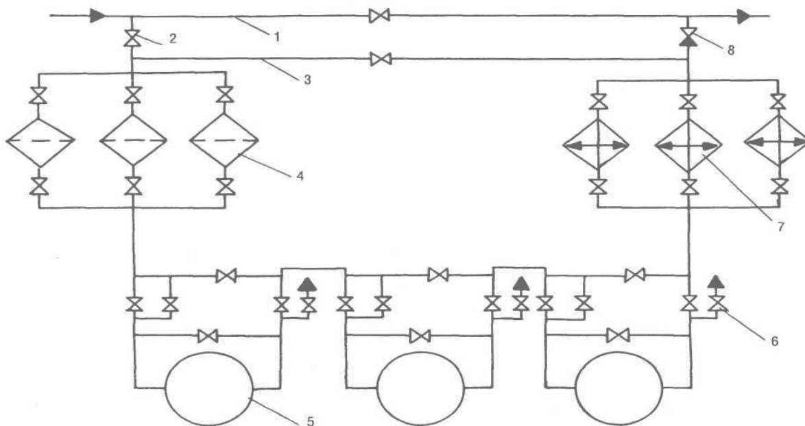
Рис.25–Технологическая схема компрессорной станции с центробежными нагнетателями: 1 – магистральный газопровод; 2 – кран; 3 – байпасная линия; 4 – пылеуловители; 5 – газоперекачивающий агрегат; 6 – продувные свечи; 7 – АВО газа; 8 – обратный клапан
