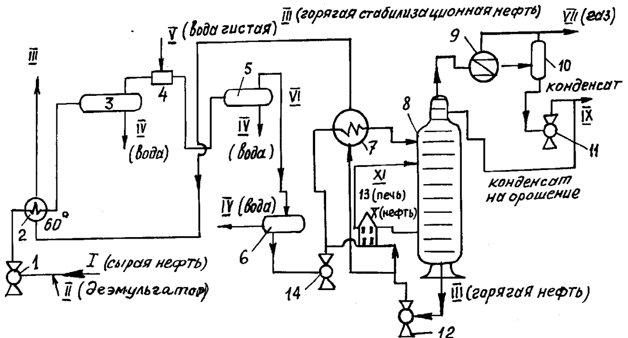
Рисунок 18—Технологическая схема УКПН:
