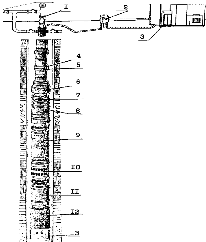
Рис.13.Схемапогружногоцентробежного насоса
