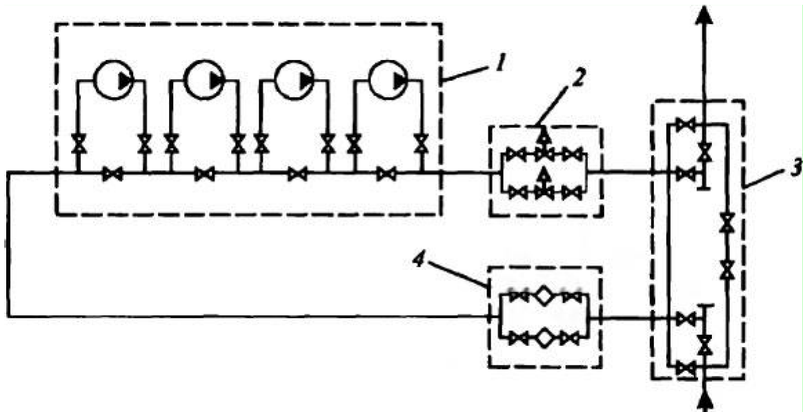
Рис.23. Технологическая схема промежуточной НПС:
