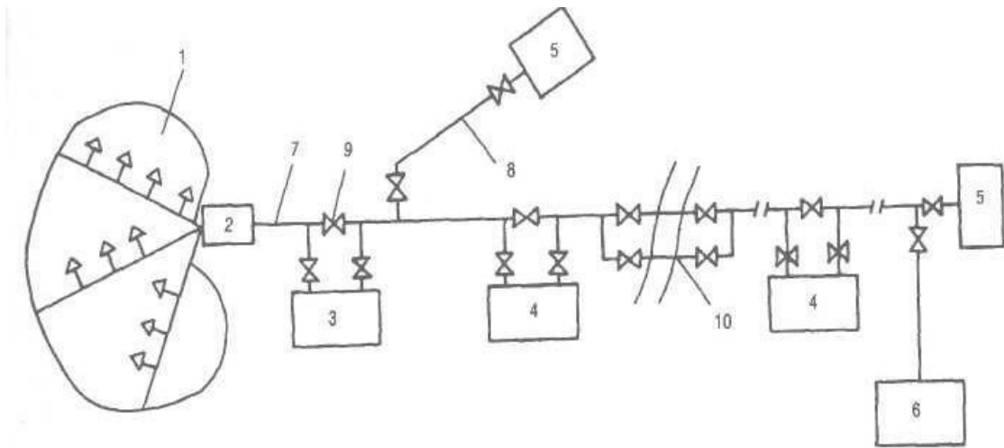
Рис.24—Схема магистрального газопровода: 1—газосборные сети; 2—промысловый пункт сбора газа; 3 — головные сооружения; 4 - компрессорная станция; 5 — газораспределительная станция; 6 — подземные хранилища; 7 — магистральный трубопровод; 8—ответвления от магистрального трубопровода; 9—линейная арматура; 10 — двухниточный проход через водную преграду.
