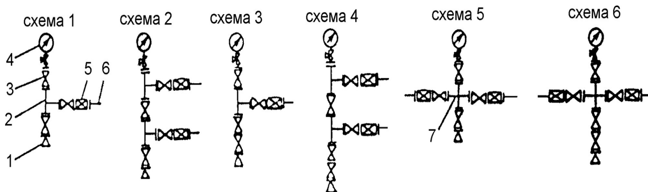
Рисунок 10 – Типовые схемы фонтанных елок: тройниковые – схемы 1, 2, 3 и 4; крестовые – схемы 5 и 6
