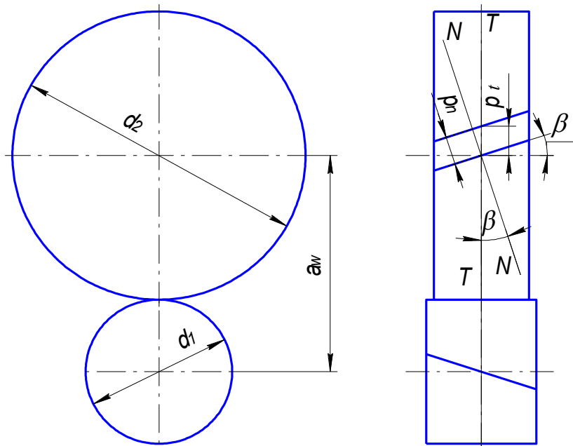
Рис. 3.2 – Косозубая передача
