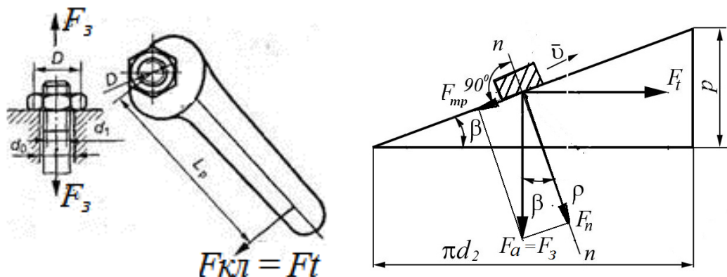
Рисунок 1- К расчету момента на ключе Рисунок 2-Силы в резьбе
