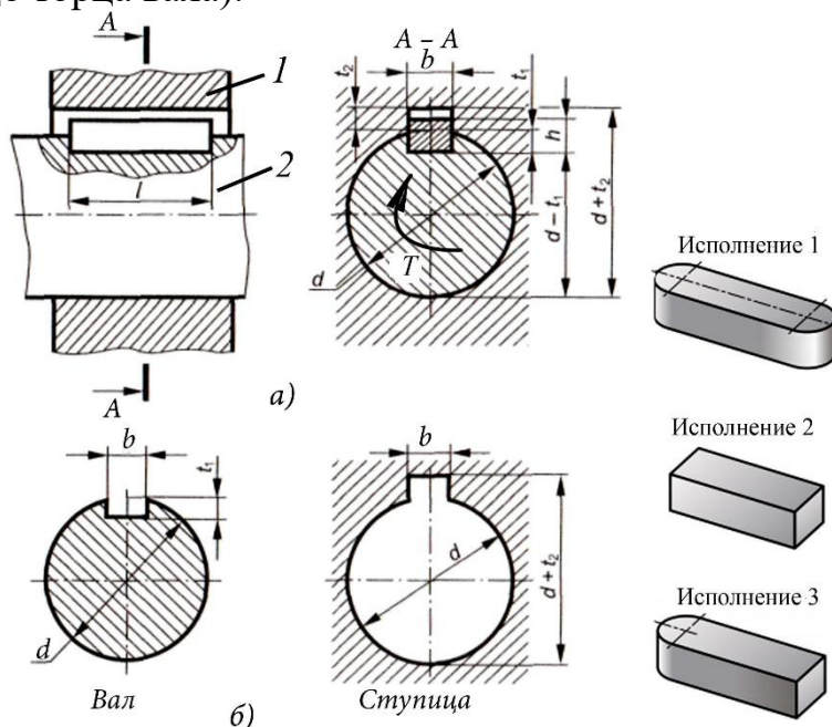
Рисунок 1 – Соединение призматической шпонкой
