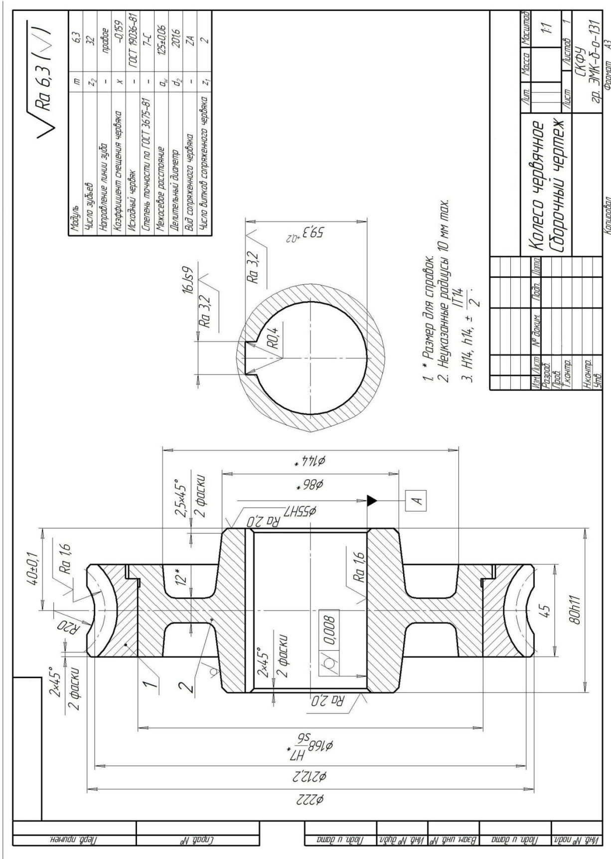
Рисунок 6 – Рабочий чертёж червячного колеса
