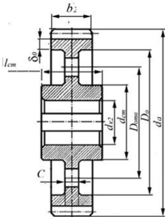
Рисунок 6 – Схема колеса
