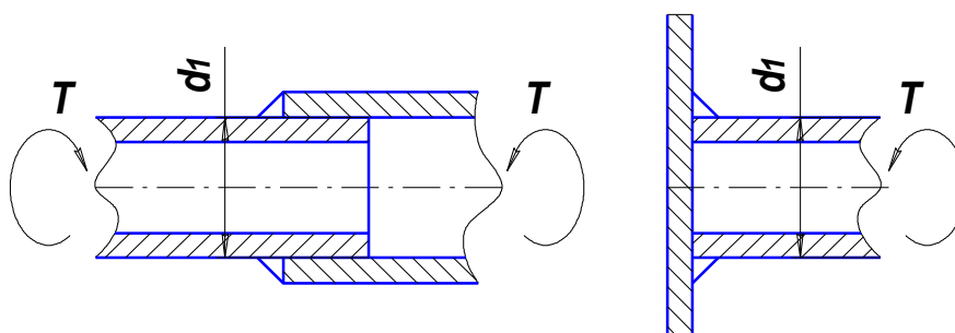
Рисунок 7.5– Стыковое соединение труб
