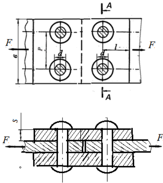
Рисунок 2-Заклепочный шов
