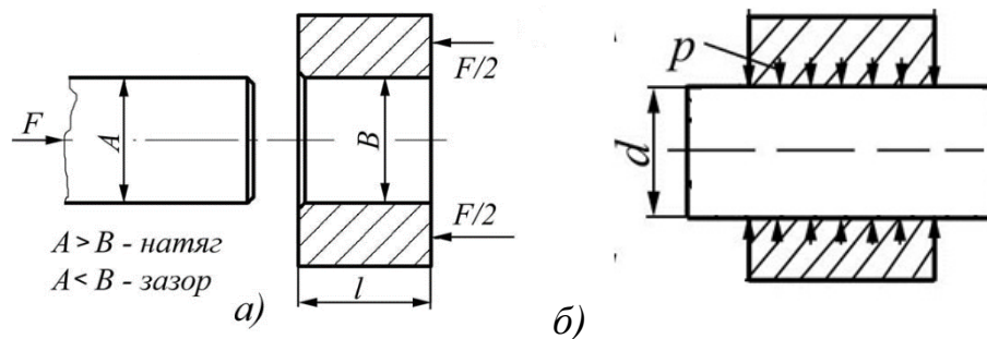
Рисунок 1 – Соединение с натягом: а) до запрессовки; б) после запрессовки
