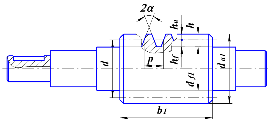
Рис. 3.1 – Червяк
