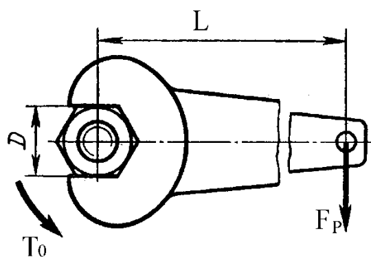
Рисунок 5 – Расчетная схема
