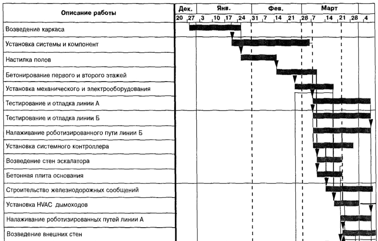
Рисунок 4.2 – Диаграмма Ганта
