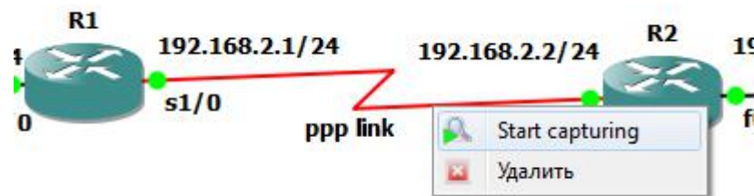
Рисунок 2 - Захват пакетов
