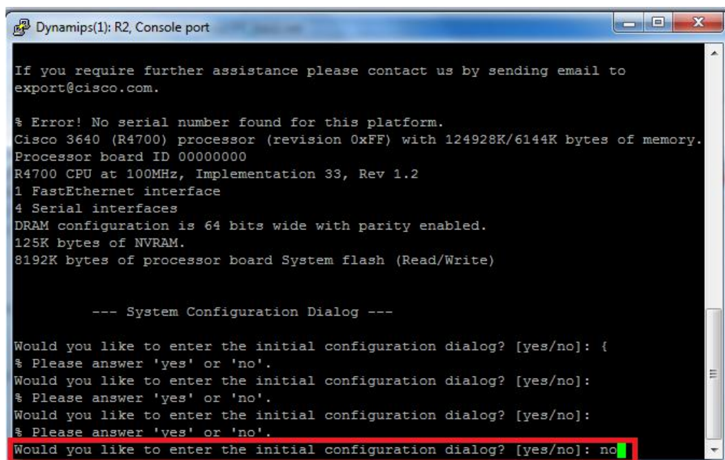
Рисунок 17 – Интерфейс командой строки маршрутизатора
