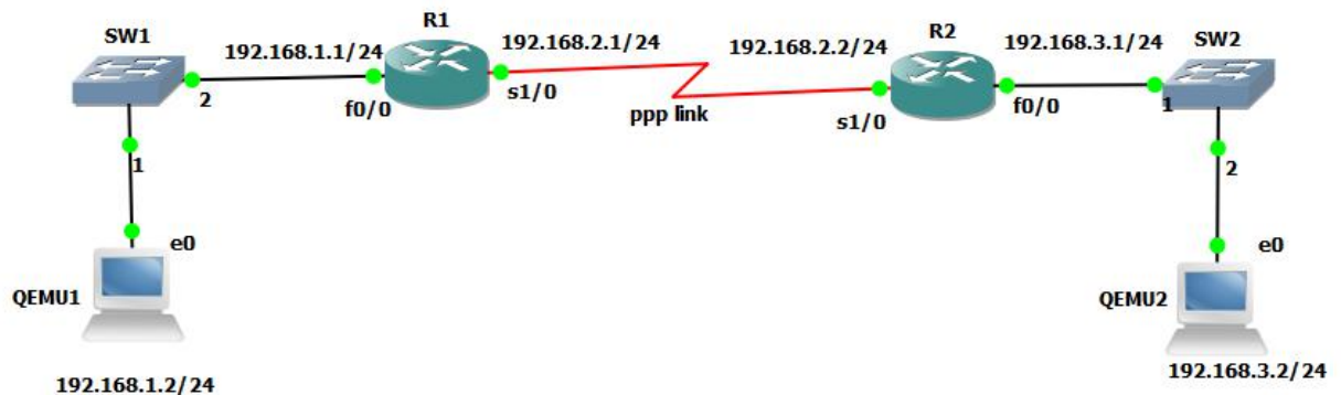
Рисунок 1 - Топология сети
