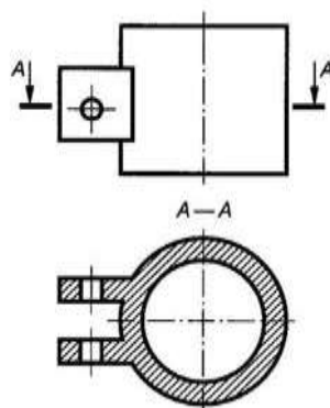
Рисунок 57– Горизонтальный разрез Рисунок 58 – Фронтальный разрез
