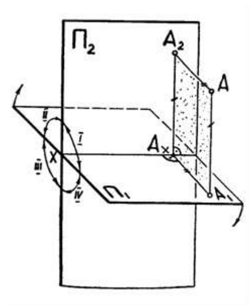
Рисунок 11 – Проекционный способ
