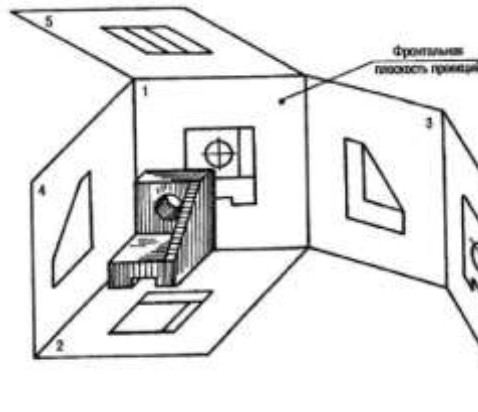
Рисунок 49 – Образование видов
