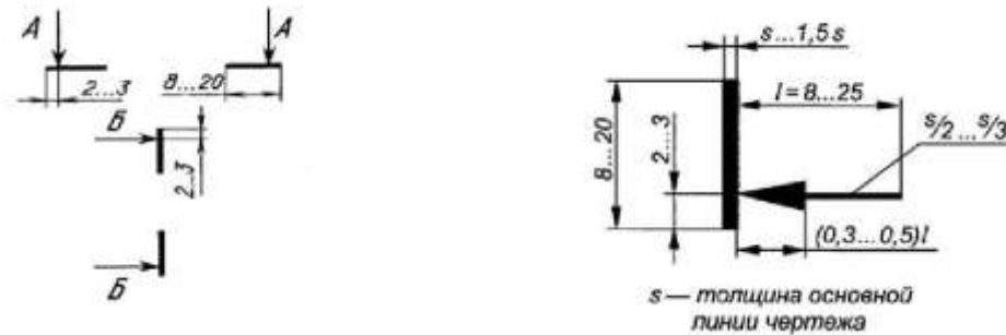
Рисунок 61 – Линия сечения
