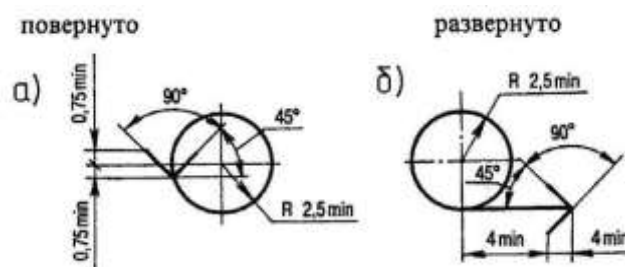
Рисунок 52 – Знаки
