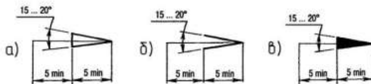
Рисунок 51 – Стрелки
