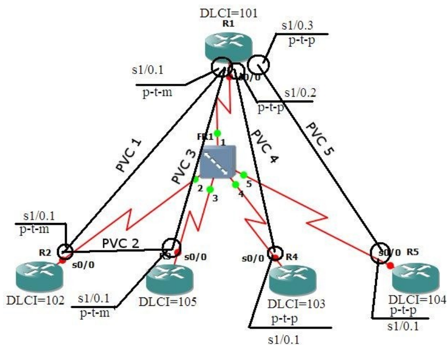
Рисунок 19 – Исследуемая топология
