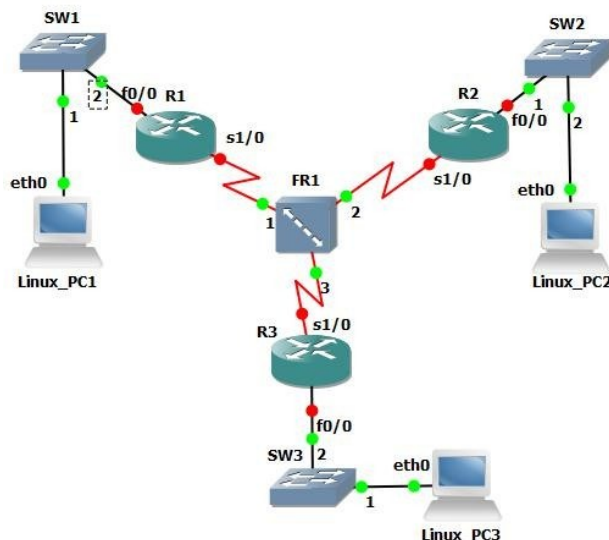
Рисунок 13 – Исследуемая топология
