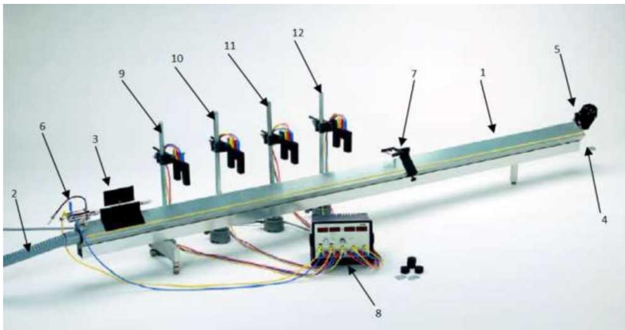
Рис.3. Экспериментальная установка для изучения равноускоренного движения
