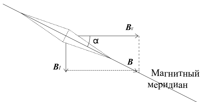
Рис.3 Магнитное склонение
