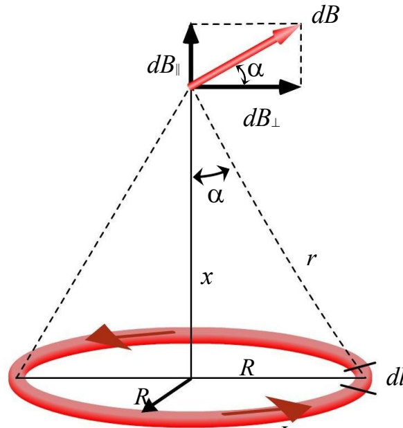
Рис. 5. Определение величины I поля оси витка
