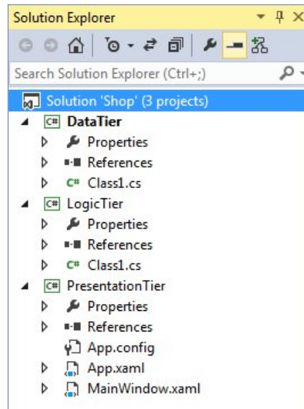
Рисунок 22.3 – Вид обозревателя проекта после добавления отдельных проектов
