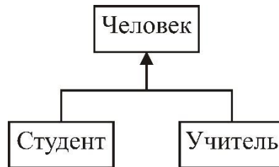
Рисунок 6.1 – Иерархия классов.
