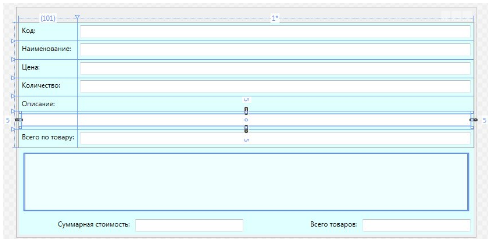
Рисунок 22.6 – Дизайн MainWindow.xaml
