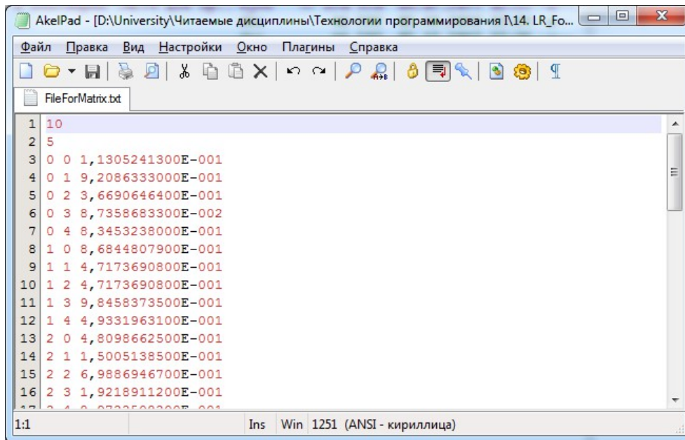
Рисунок 14.7 – Результирующий файл
