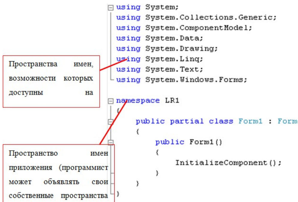
Рисунок 8.3 –Листинг Form1.cs
