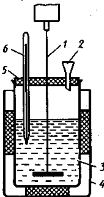
Рисунок 19. Калориметрическая установка: 1- мешалка; 2 - воронка; 3 - калориметрический (внутренний) стакан; 4 - наружный стакан; 5 - крышка из пенопласта; 6 - термометр.
