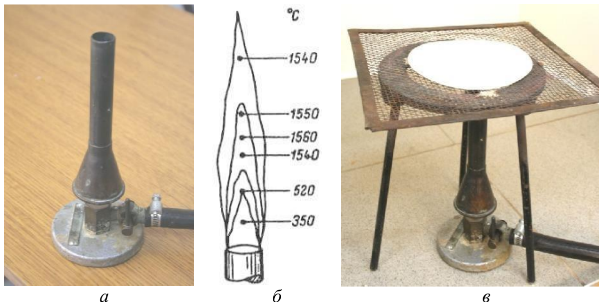
Рисунок 12. Горелка Теклю (а), распределение температуры в пламени газовой горелки (б) и штатив-подставка с асбестовой сеткой над горелкой (в)
