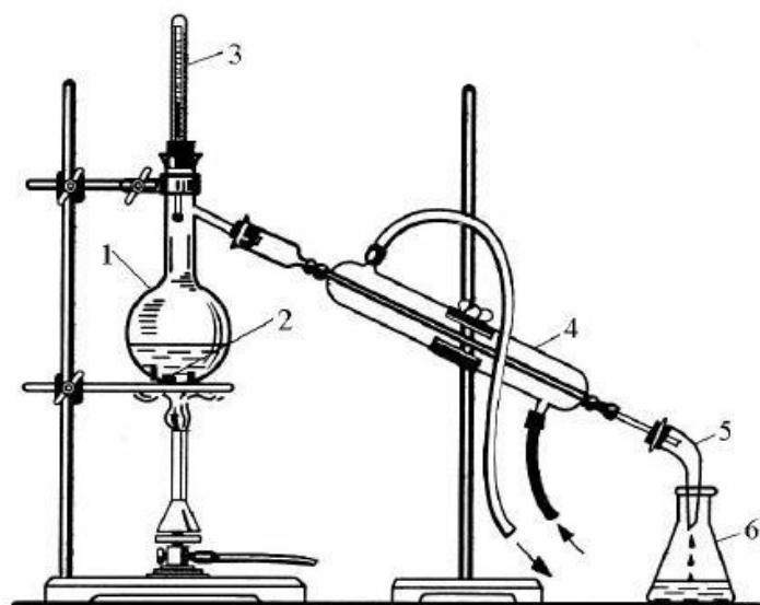
Рисунок 16. Прибор для простой перегонки
