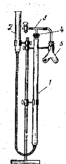
Рисунок 18. Прибор для определения эквивалента металла: 1- бюретка на 100 мл; 2 - уравнительный сосуд; 3 - стеклянный тройник с каучуковой трубкой и краном; 4 - каучуковая пробка; 5 - склянка Оствальда с пробкой.
